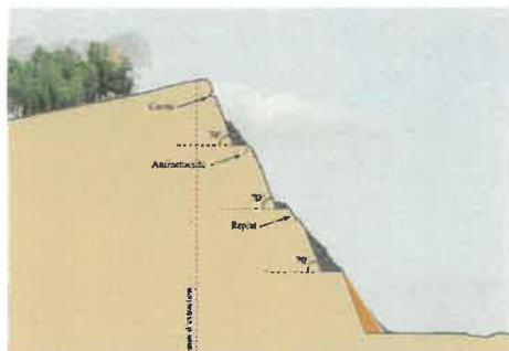
Réaménagement des fronts de taille
