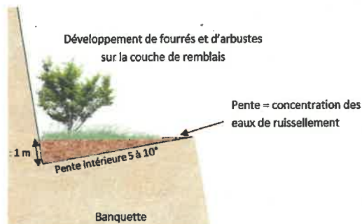
Réaménagement des banquettes
