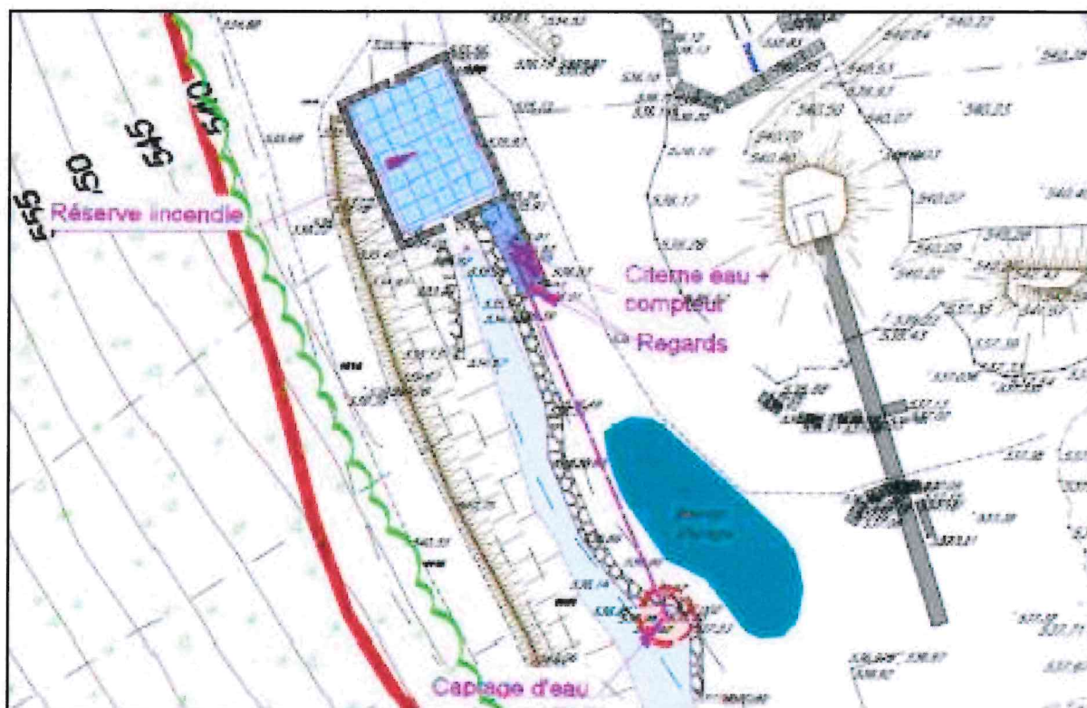
Fig.16. Vue en plan du bassin d'orage
