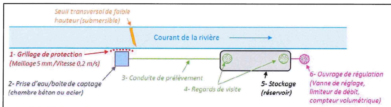
Schéma de principe de la prise d'eau
