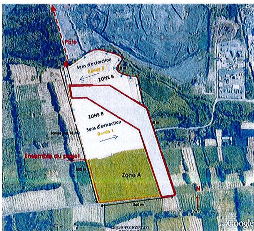
Plan de phasage, zone B
