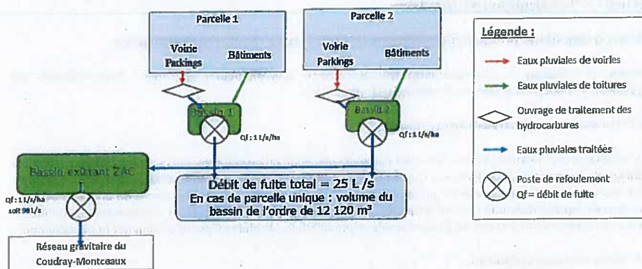
Schéma de principe de la gestion des eaux pluviales sur le site de l'extension de la ZAC « Les Haies Blanches »
