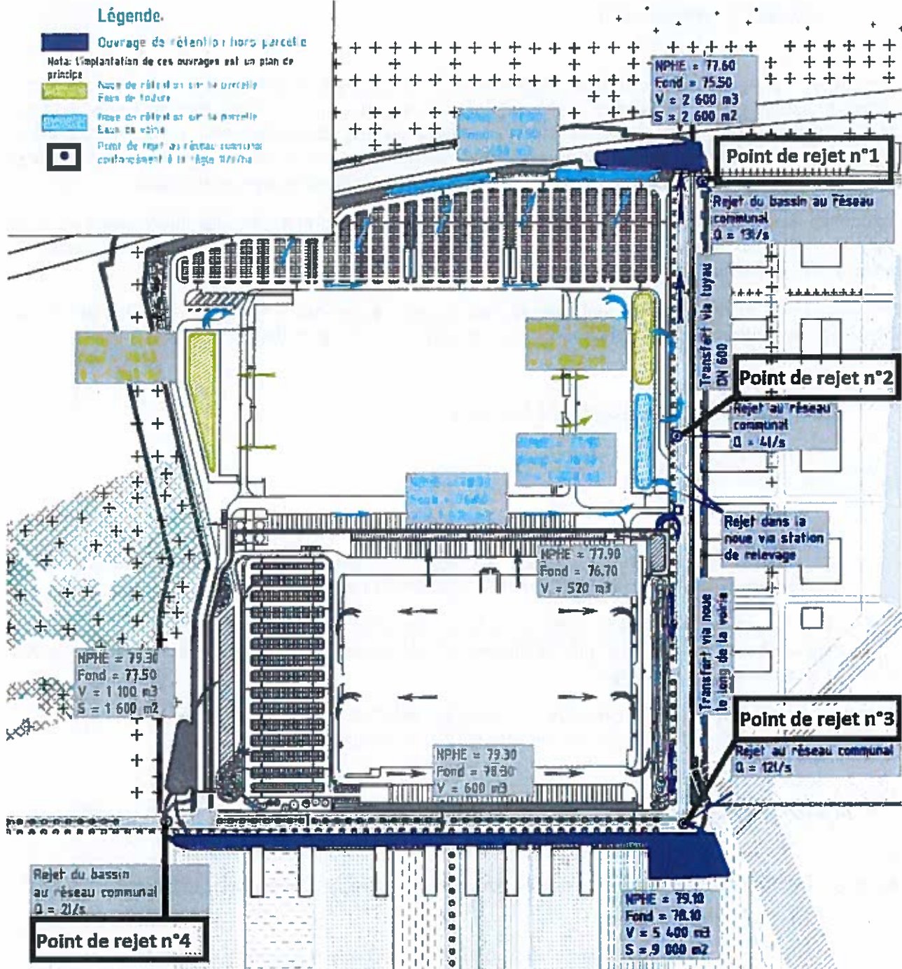
Figure 2 : Schéma des réseaux d'eaux pluviales
