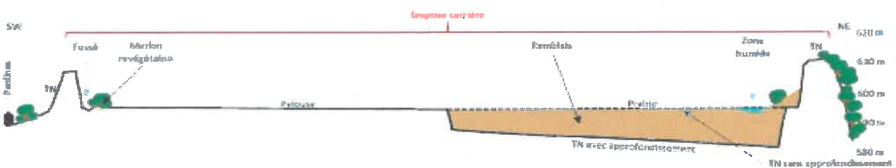
Figure 16 : profil topographique de principe, après réaménagement - coupe schématique longitudinale SW/NE
