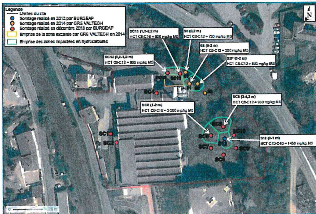
Figure 13 : Emprises horizontales des zones impactées en hydrocarbures volatils
