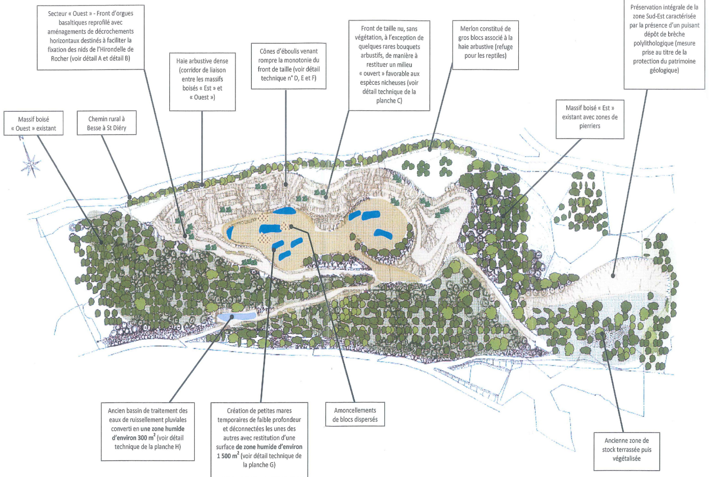
PLAN PROJET DE LA REMISE EN ETAT (Echelle : 1/2000)
