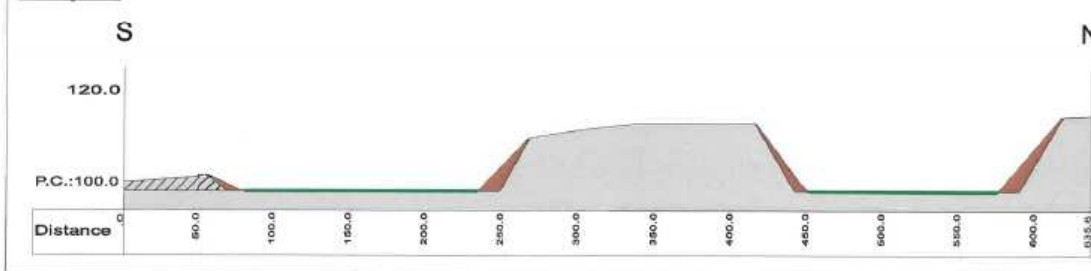
Coupe 3
