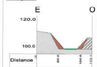
Coupe 2
