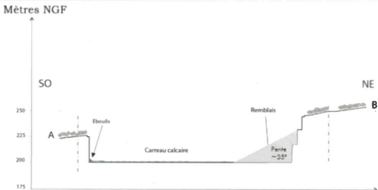
Coupe AB de l'état final de la partie Nord Est du site
