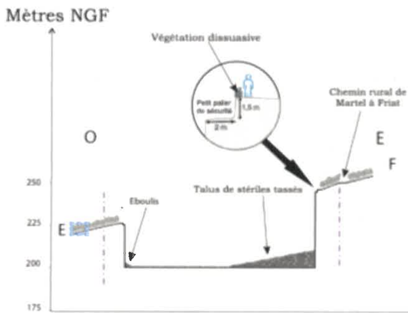
Coupe EF de l'état final du reste du site
