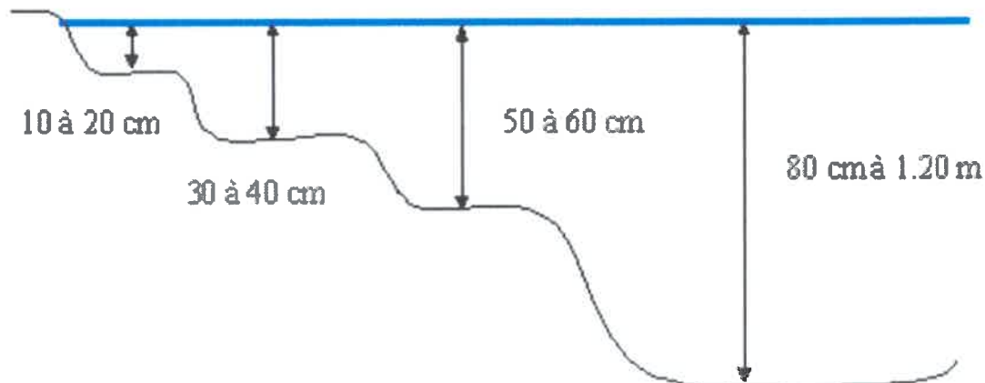
Profil de la mare à créer
