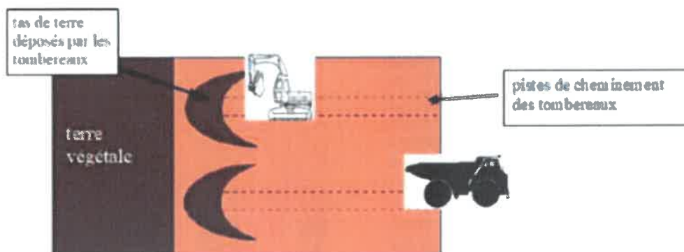
Exemple de réaménagement du sol par cheminement unique des tombereaux (extrait étude agro-pédologique de la Chambre d'Agriculture de l'Isère)
