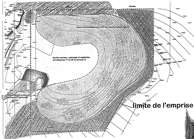
Schéma du réaménagement sur fond topographique à l'échelle du 1/2000
