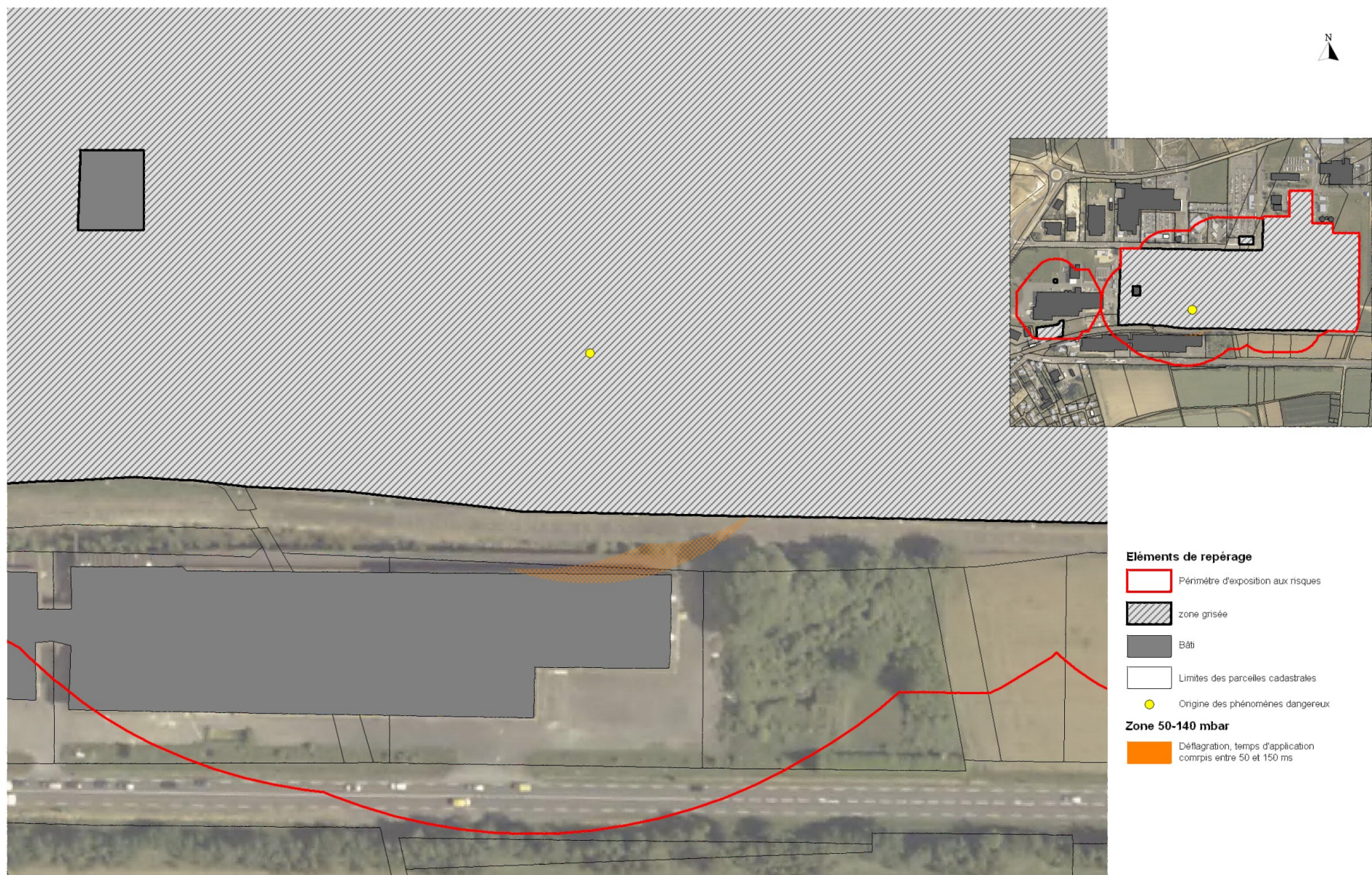
PPRT BASF Coatings à Breuil-le-Sec Carte n°1-4 bis "Surpression maximale de 140 mbar déflagration"
