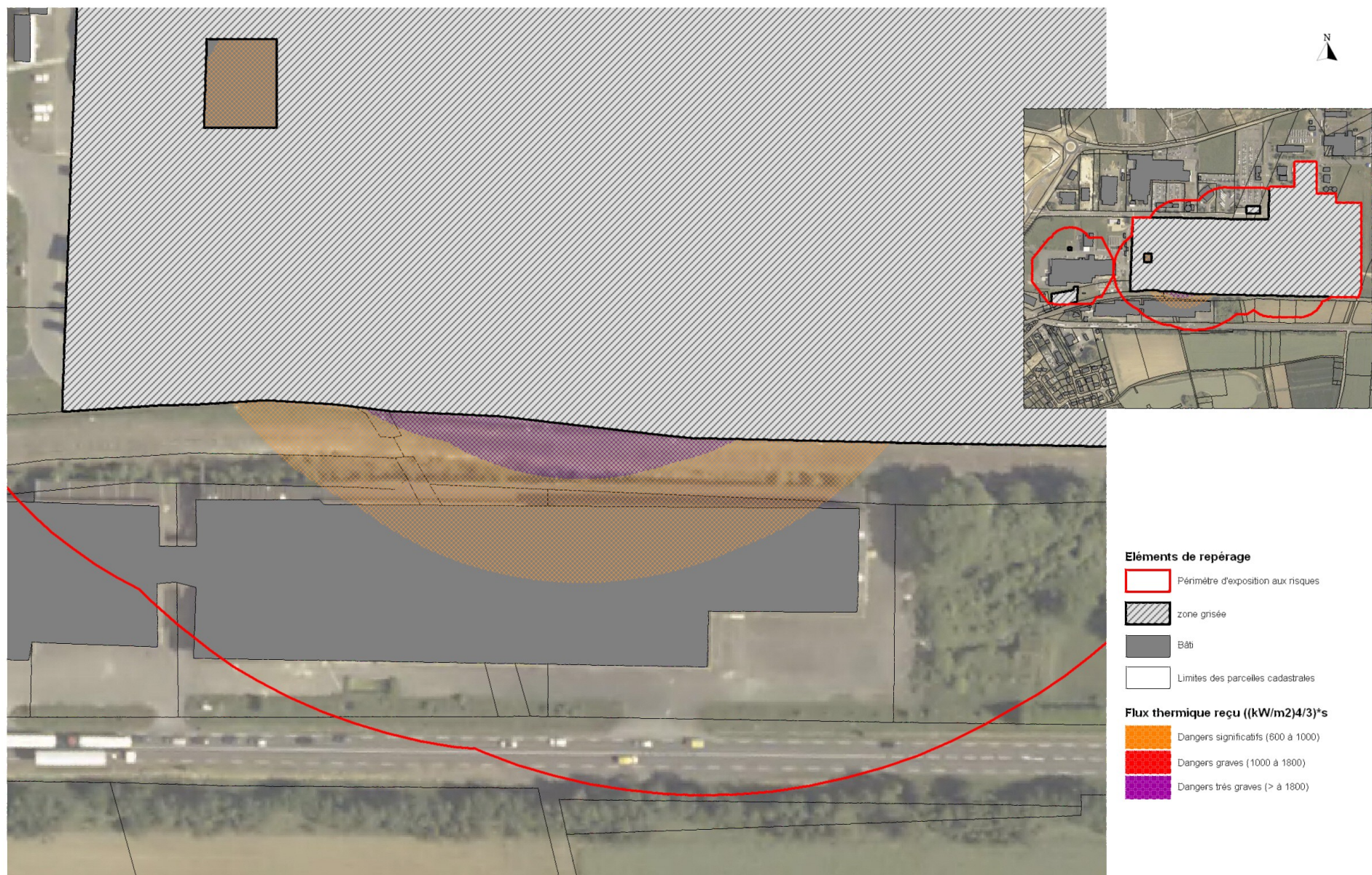
PPRT BASF Coatings à Breuil-le-Sec Carte n°2-2 "Intensité thermique transitoire de type boule de feu"
