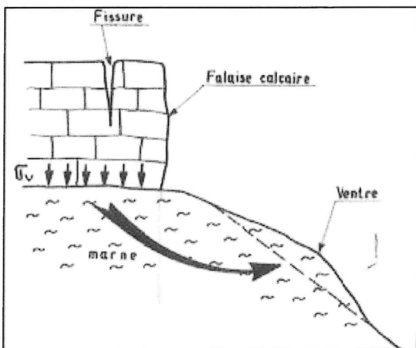
Illustration 4: Fluage d'après Philipponnat & al. (note BRGM)
