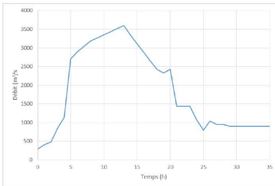
Illustration 37 : Hydrogramme de la crue de 1940 de la Têt en amont immédiat de Perpignan
