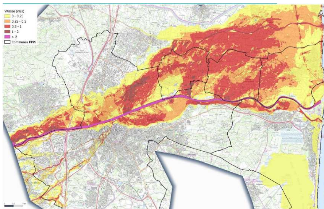
Illustration 43 : Vitesses d'écoulement de la crue de référence de la Têt
