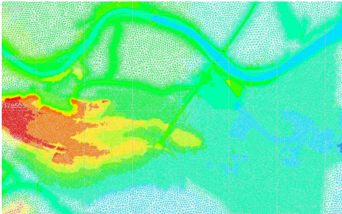
Illustration 36 : Extrait du maillage du modèle Têt et affluents
