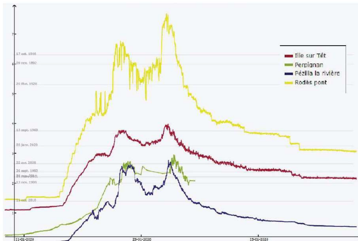
Illustration 31 : Limnigrammes de crue de la Têt
