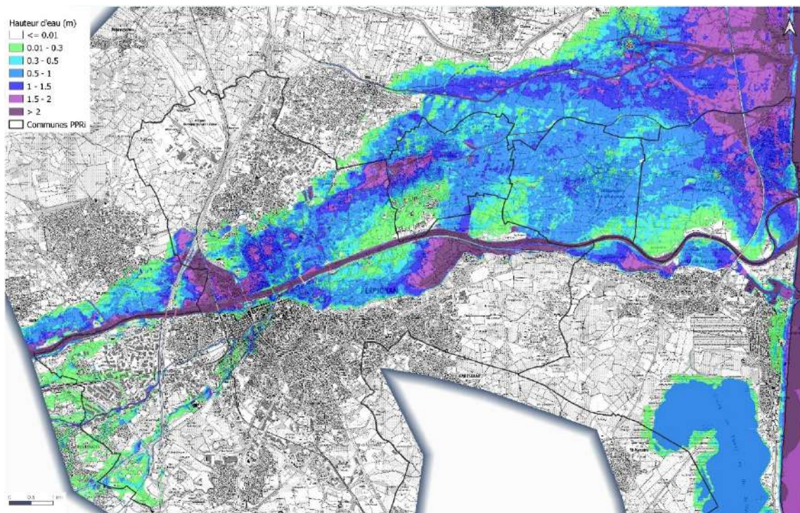
Illustration 38 : Hauteurs d'eau pour la crue de référence de la Têt (crue de type 1940)
