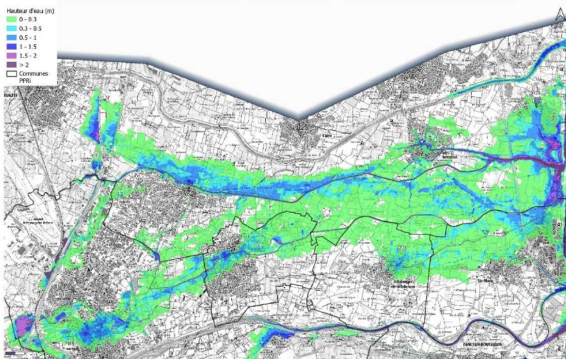
Illustration 40 : Hauteurs d'eau pour les débits de référence (centennaux) des cours d'eau rive gauche
