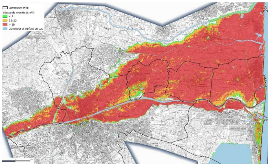
Illustration 42 : Vitesses de montée de l'eau de la crue de référence de la Têt
