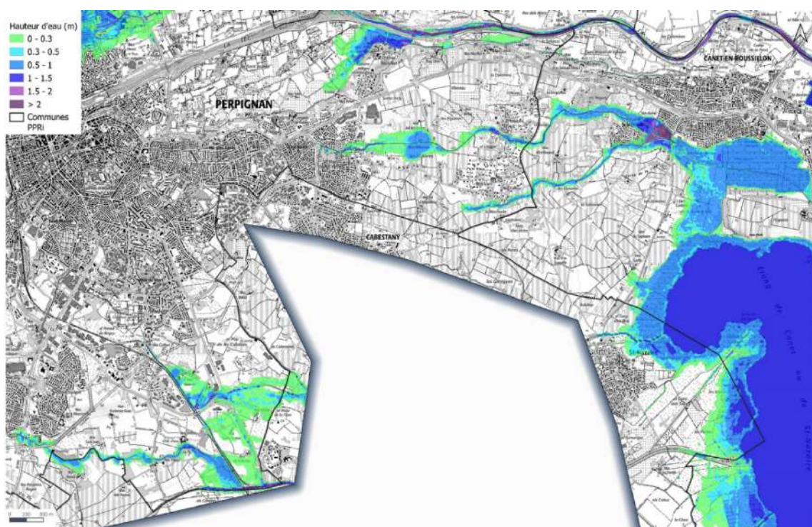
Illustration 41 : Hauteurs d'eau pour les débits de référence (centennaux) des cours d'eau rive droite
