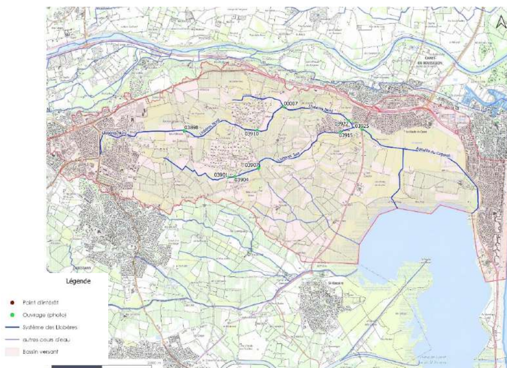
Illustration 17 : Système hydrographique des Llobères
