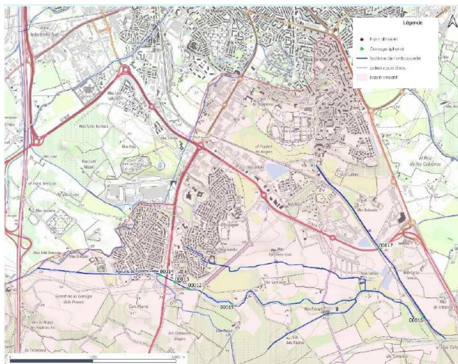
Illustration 18 : Système hydrographique de Fontcouverte
