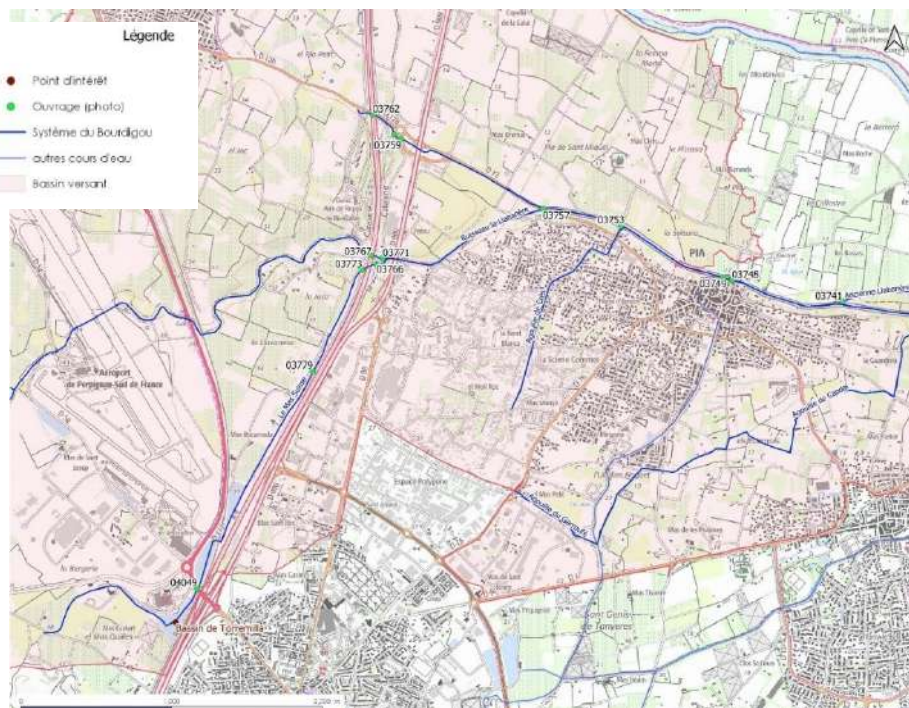
Illustration 15 : Cours d'eau amont du système hydrographique Llabanère / Bourdigou impactants la commune de Perpignan
