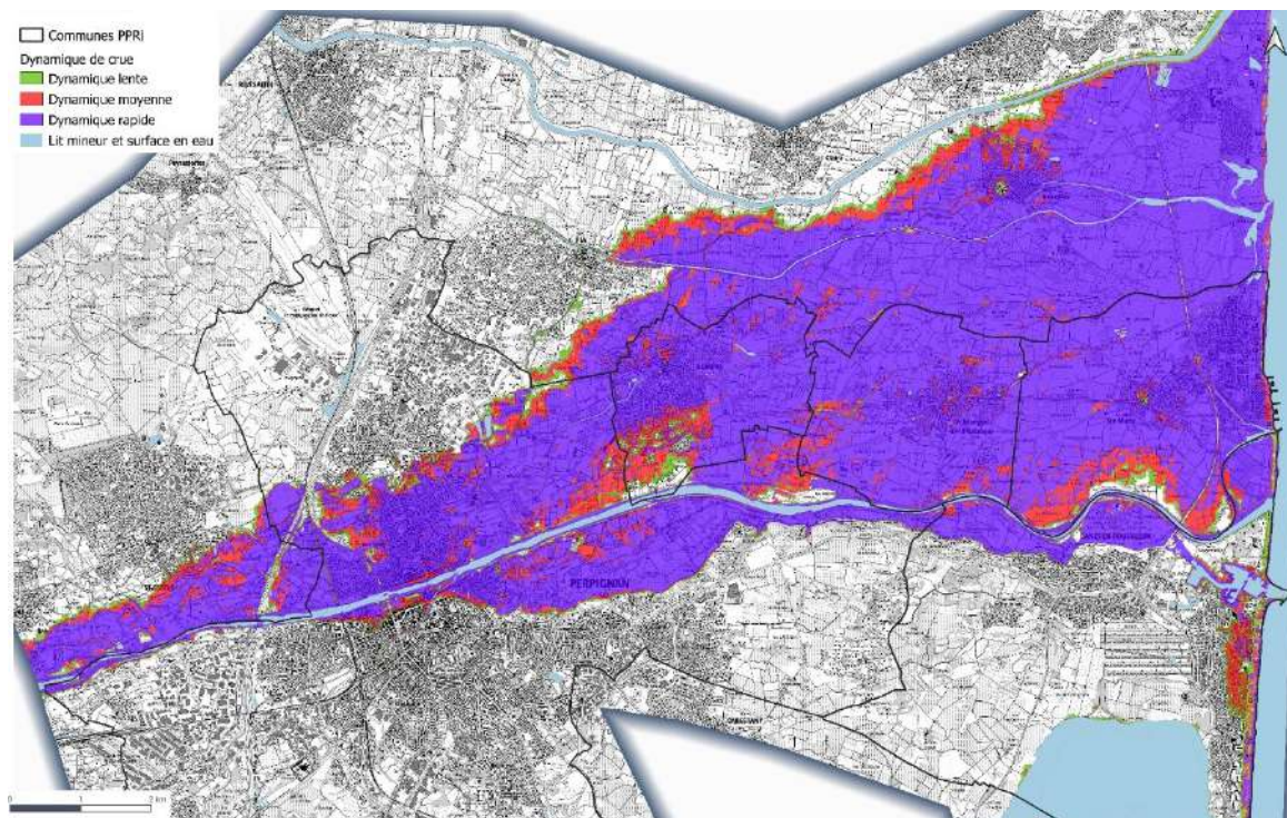
Illustration 44 : Dynamique de la crue de référence de la Têt
