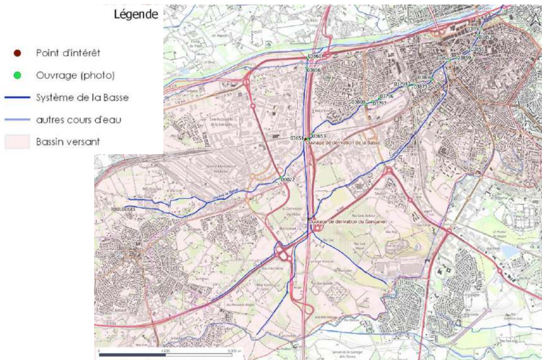
Illustration 16 : Système hydrographique Basse et Ganganeil sur la commune de Perpignan
