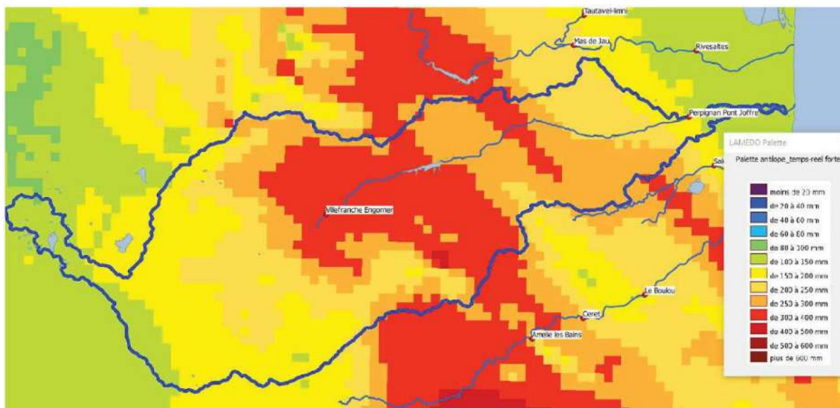
Illustration 29 : Image radar des pluies entre le 20 et le 25 janvier 2020
