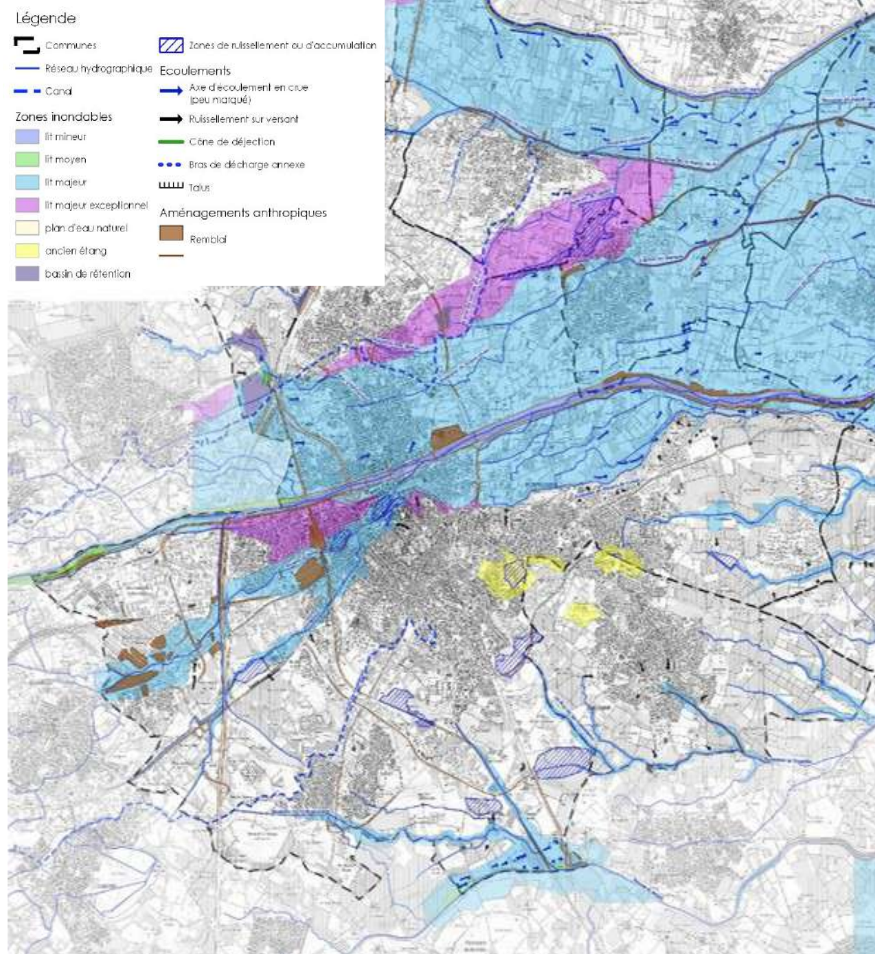
Illustration 34 : Cartographie de l'hydrogéomorphologie sur le secteur de Perpignan
