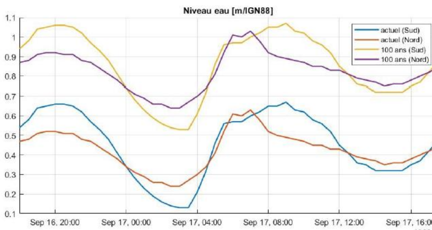
Figure 38 : signaux temporels du niveau d’eau pour les scénarios de référence actuel et 2100, basés sur l’évènement historique de l’ouragan Hugo
