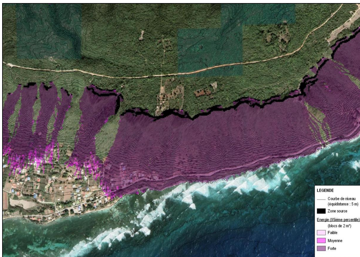
Figure 27 : Extrait des résultats de la modélisation trajectographique 3D (énergie au 95ième percentile) sur La Désirade [Source : Ginger CEBTP]
