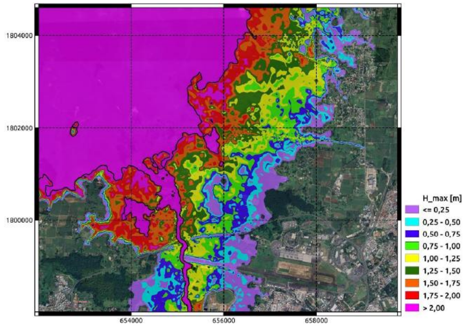
Figure 46 : Scénario de référence 2100 (Hugo) : hauteurs d'eau maximales calculées sur le bassin de risque du Grand Cul-de-Sac Marin.
