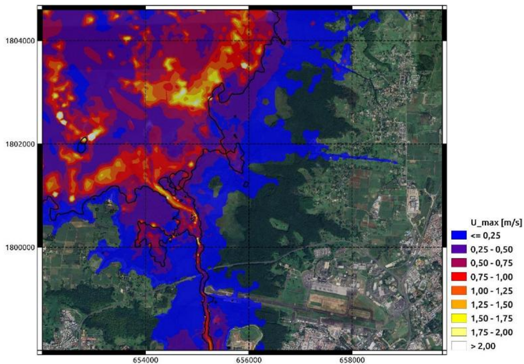
Figure 41 : Scénario de référence actuel (Ouragan 1928) : vitesse maximale des courants maximaux calculées sur le bassin de risque du Grand Cul-de-Sac Marin.
