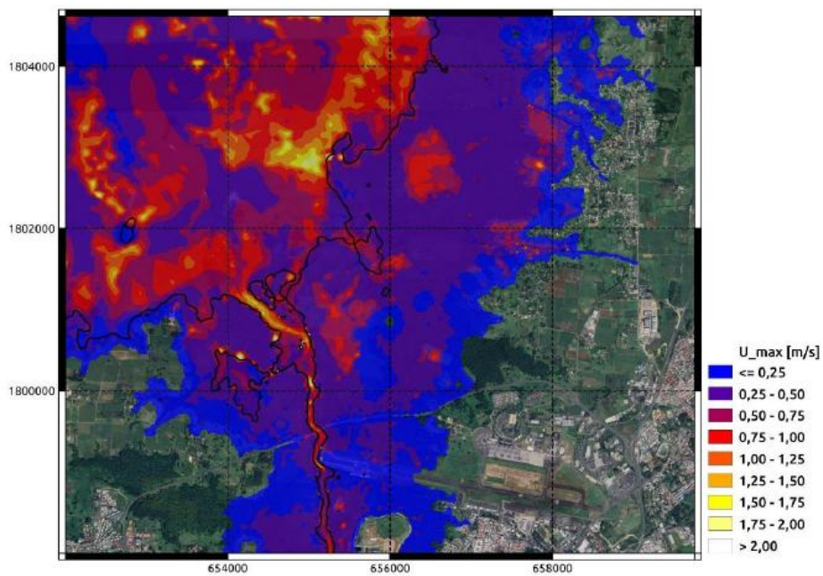
Figure 47 : Scénario de référence 2100 (Hugo) : vitesses des courants maximums calculées sur le bassin de risque du Grand Cul-de-Sac Marin.
