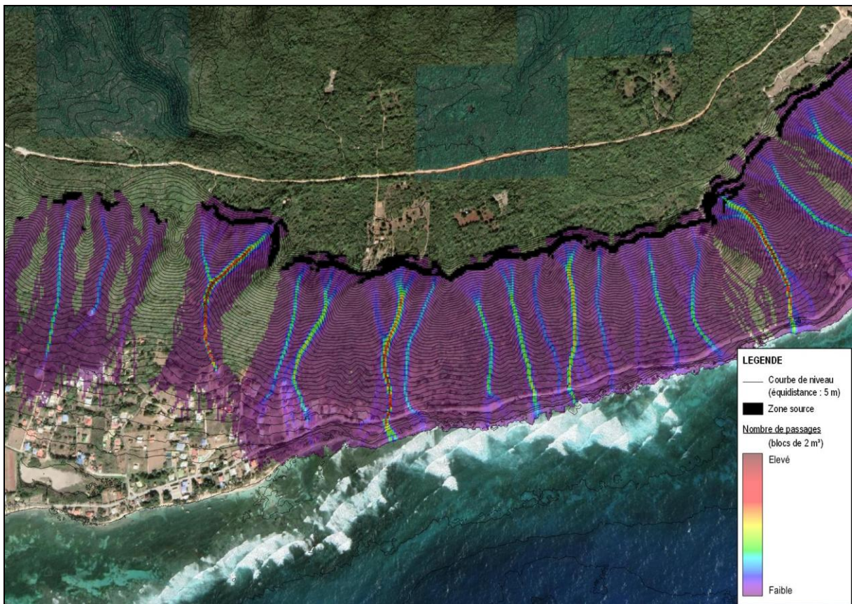
Figure 26 : Extrait des résultats de la modélisation trajectographique 3D (nombre de passages) sur La Désirade [Source : Ginger CEBTP]
