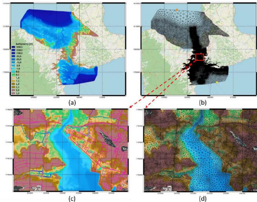
Figure 36 : Site du Petit Cul-de-sac marin : (a) : emprise spatiale du domaine de calcul et données topo-bathymétriques ; (b) Maillage de calcul et point de forçage (en orange et jaune) ; (c) topo-bathymétrie et lignes de contraintes (violet et bleu) dans la vill
