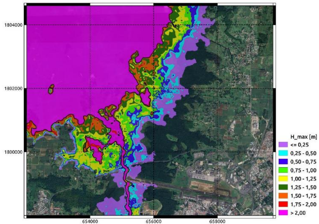
Figure 42 : scénario de référence actuel (Hugo) : hauteurs d'eau maximales calculées sur le bassin de risque de du Grand-Cul-de-Sac Marin.
