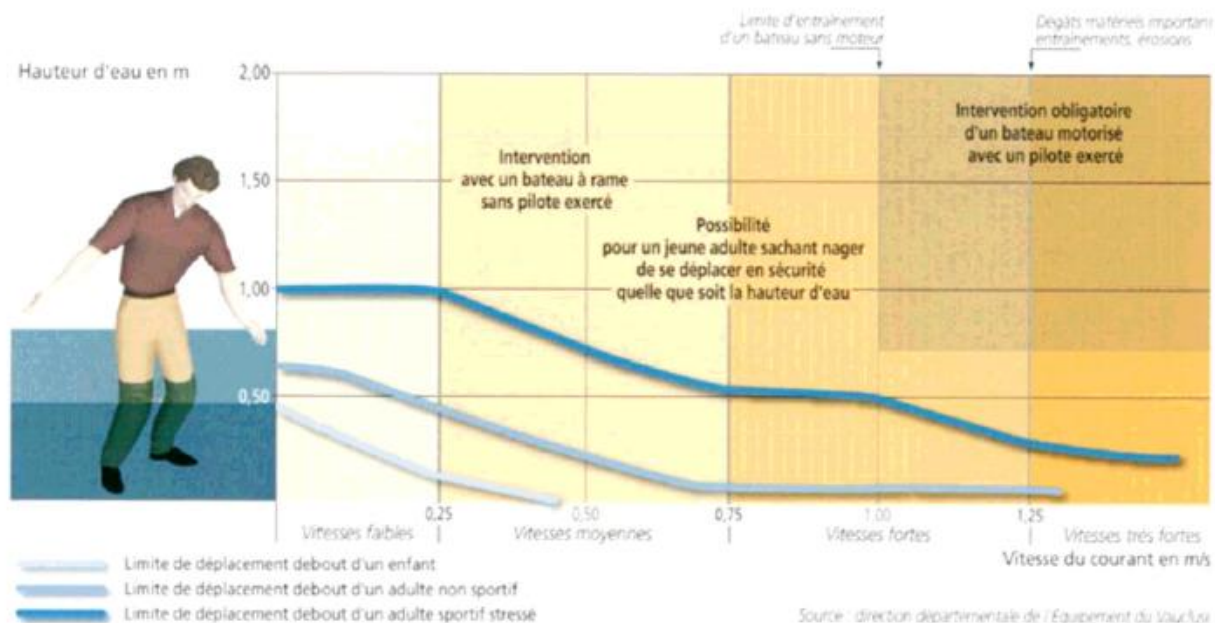
Figure 24 : Déplacement d'une personne en fonction de la hauteur d'eau et de la vitesse d'écoulement. Source : Guide méthodologique pour l'élaboration des PPR
