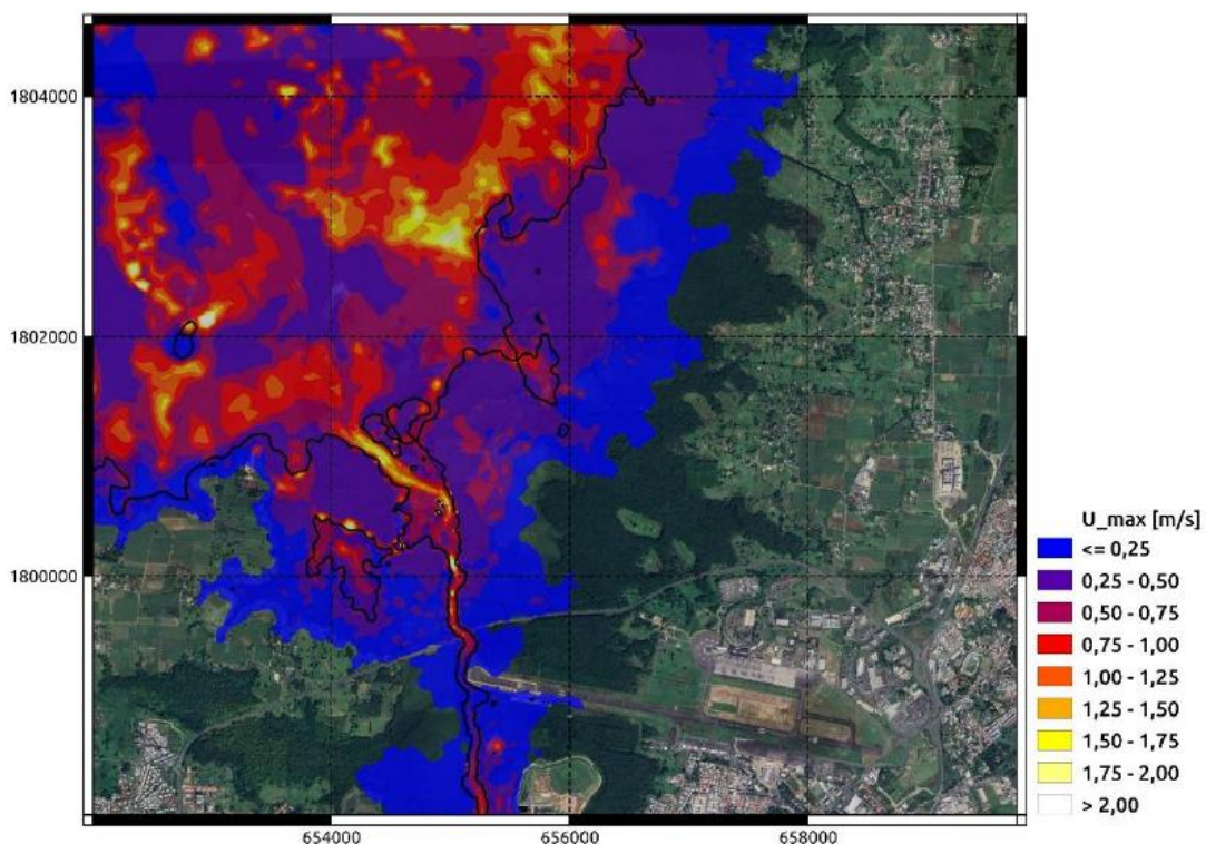
Figure 43 : Scénario de référence actuel (Hugo) : vitesses des courants maximums calculées sur le bassin de risque du Grand-Cul-de-Sac Marin.
