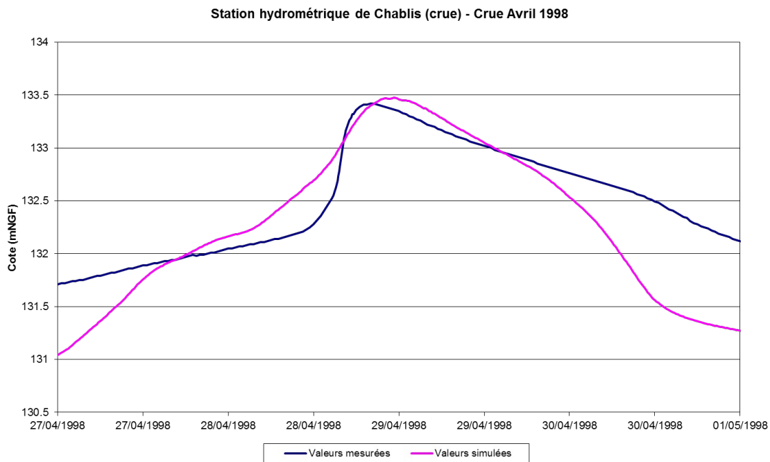
Comparaison des hauteurs d'eau mesurées et simulées à la station de Chablis (crue) – Crue d'avril 1998
