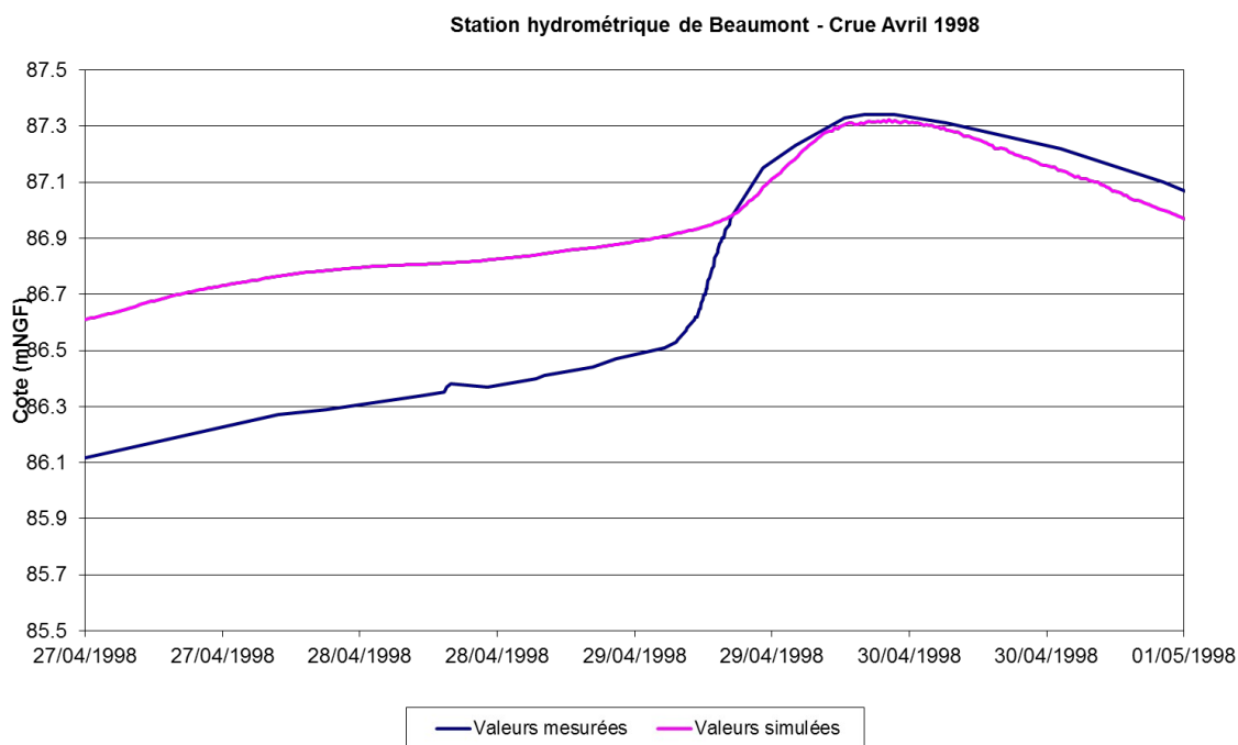
Comparaison des hauteurs d'eau mesurées et simulées à la station de Beaumont – Crue d'avril 1998
