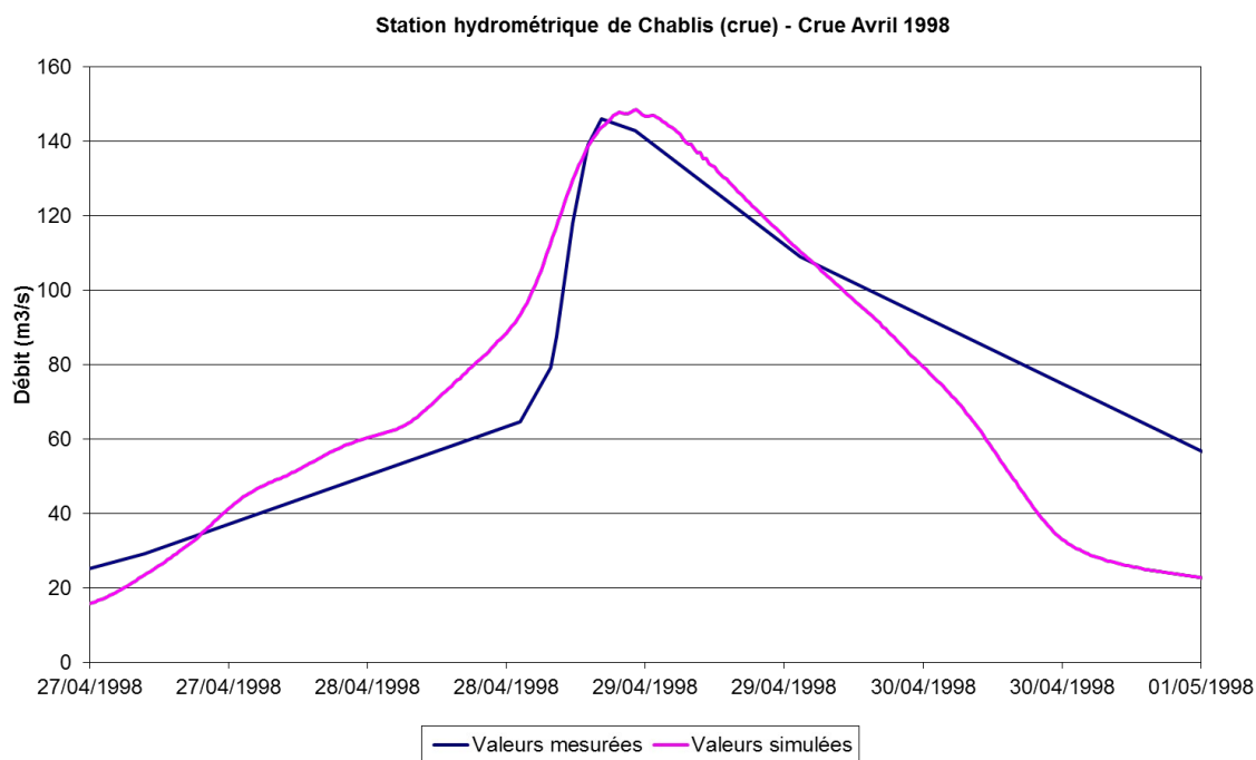
Comparaison des débits mesurés et simulés à la station de Chablis (crue) – Crue d'avril 1998
