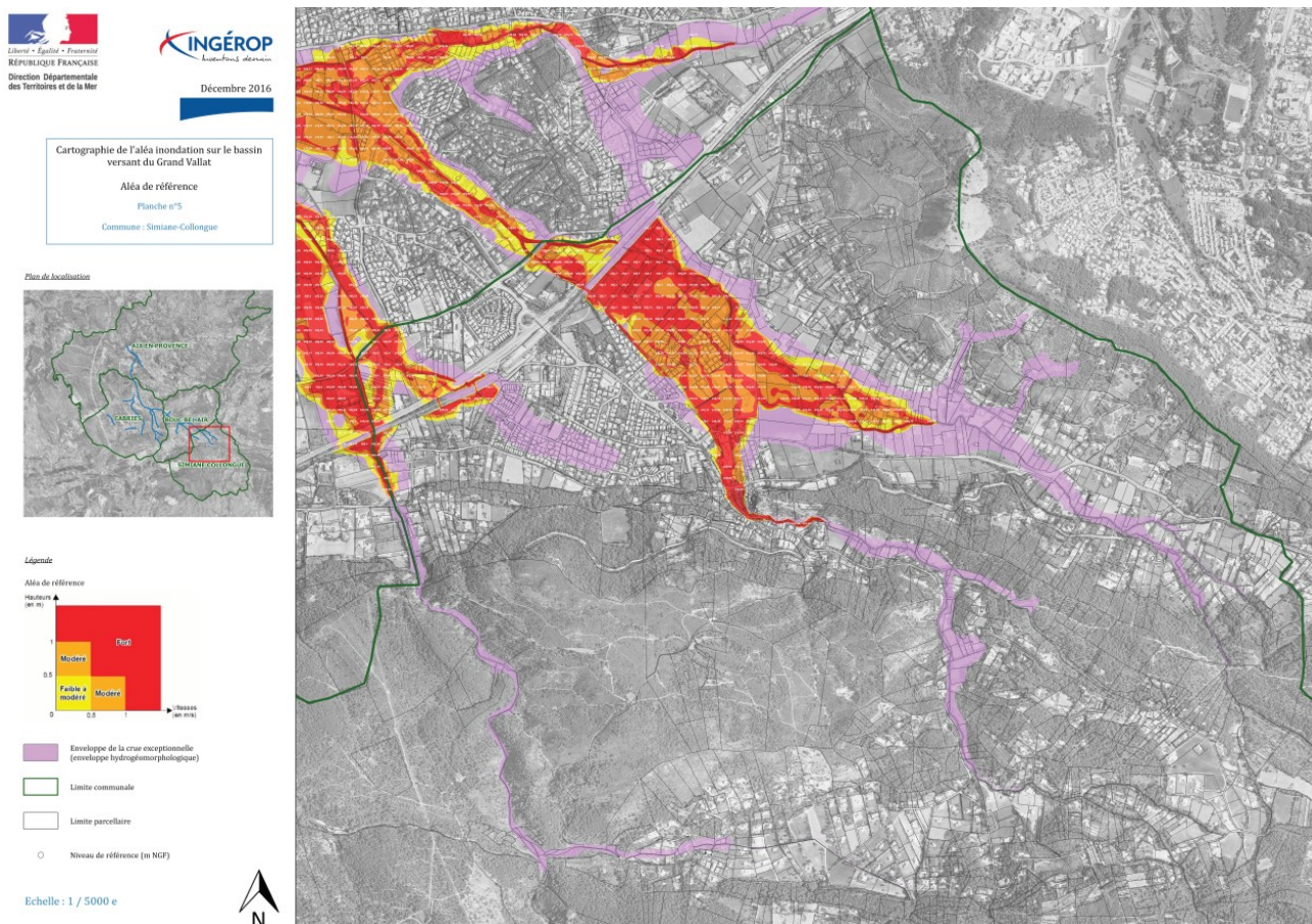
Figure 28 : Cartographie de l'aléa (DDTM-INGEROP-2017)
