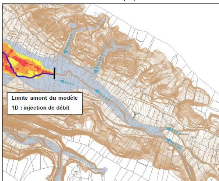
Figure 33 : Organisation des écoulements – Vallat de Babol – secteur 1 (DDTM-INGEROP-2018)
