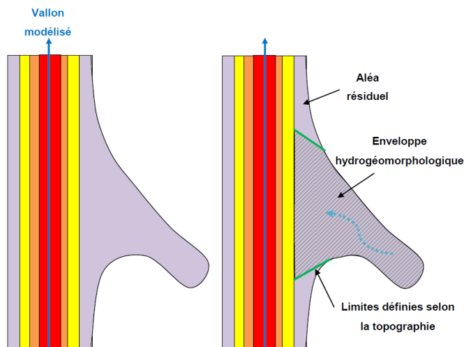
Figure 31 : Exemple d'aléa indifférencié représentant un axe d'écoulement latéral (DDTM-INGEROP-2018)
