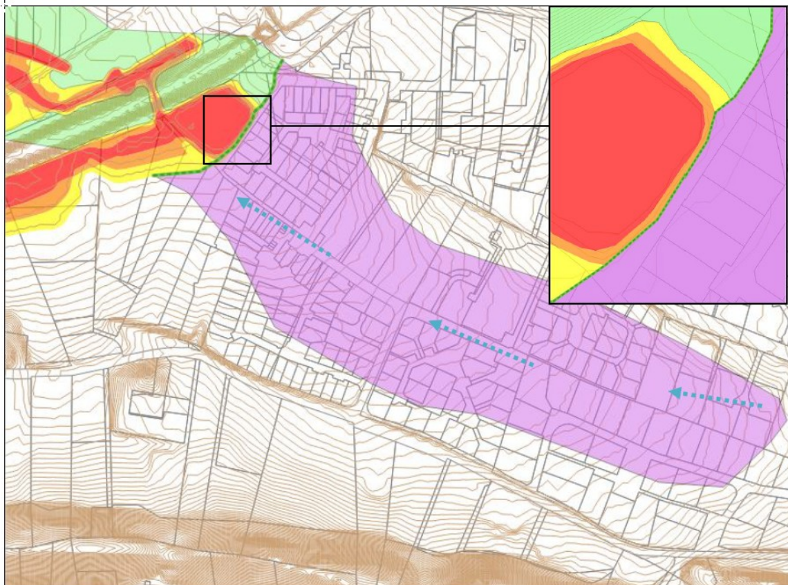
Figure 40 : Précision de l'aléa : Vallat de Rajol (DDTM-INGEROP-2018)
