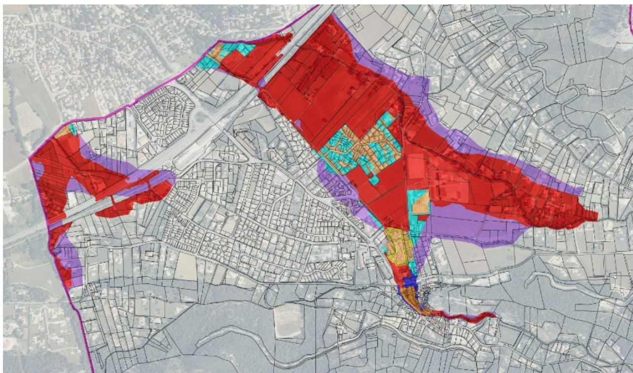
Figure 54 : Zonage réglementaire du présent PPRi sur la commune de Simiane-Collongue
