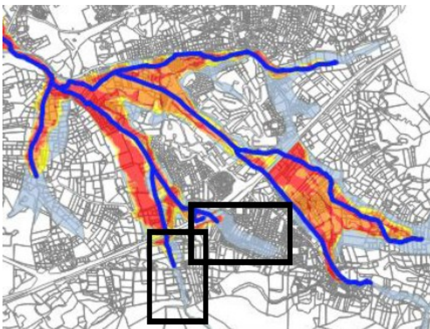
Figure 39 : Localisation des secteurs étudiés le long des Vallat de Rajol et Vallat des Tilleuls (DDTM-INGEROP-2018)
