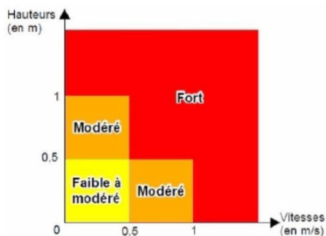
Figure 24 : Grille d'aléa (Source DDTM 13)
