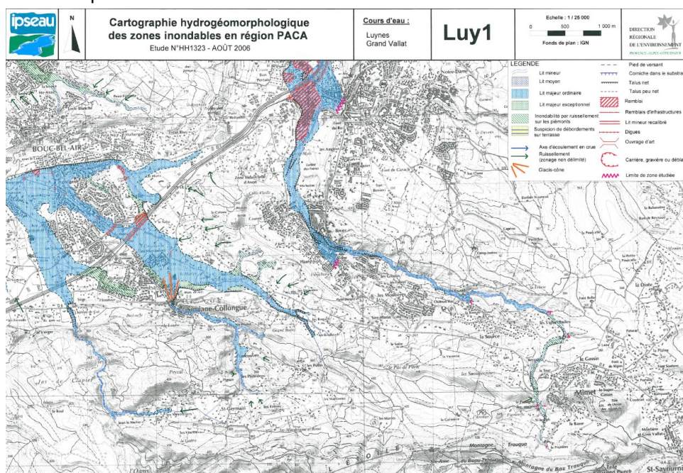
Figure 12 : Cartographie hydrogéomorphologique des zones inondables en région PACA, Cours d'eau du Grand Vallat (Source IPSEAU 2004)
