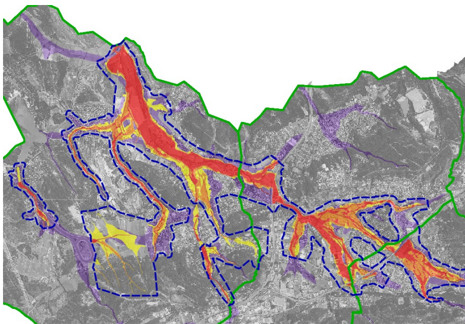
Figure 25 : Extrait du Porter à connaissance inondation sur les communes de Bouc Bel Air, Cabriès et Simiane-Collongue du 6 octobre 2017.
