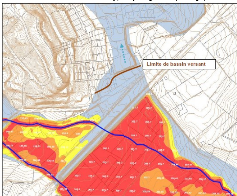
Figure 35 : Organisation des écoulements – Vallat de Babol – secteur 2 (DDTM-INGEROP-2018)
