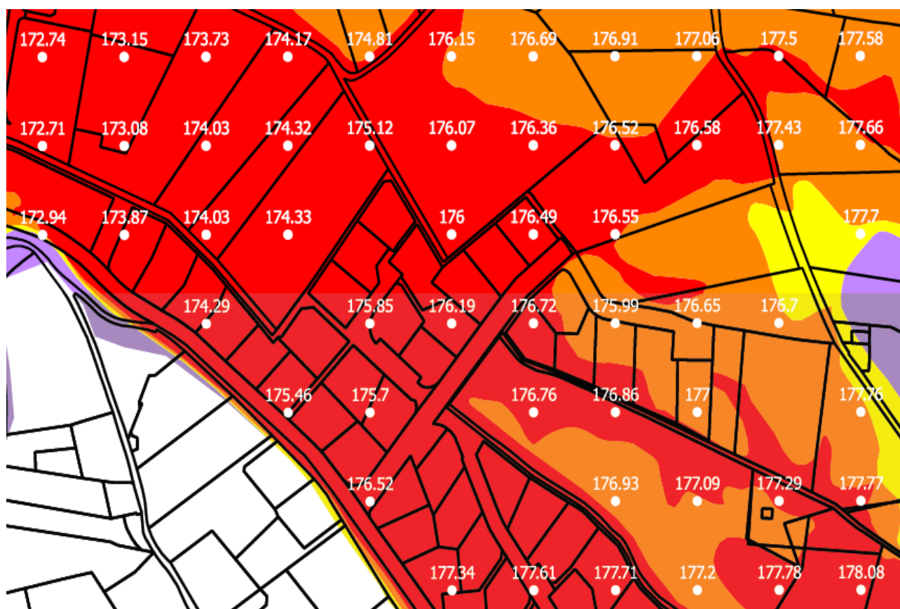
Figure 55 : Extrait de la carte des Plus Hautes Eaux (PHE) du PPRi de la commune de Simiane-Collongue
