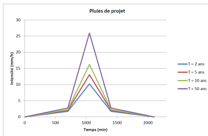
Figure 15 : Les pluies de projet d'occurrence 2, 5, 10 et 50 ans.
