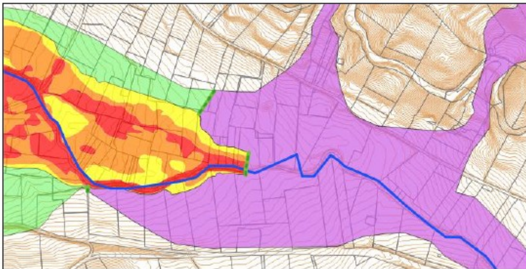
Figure 34 : Précision de l'aléa : Vallat de Babol – Secteur 1 (DDTM-INGEROP-2018)
