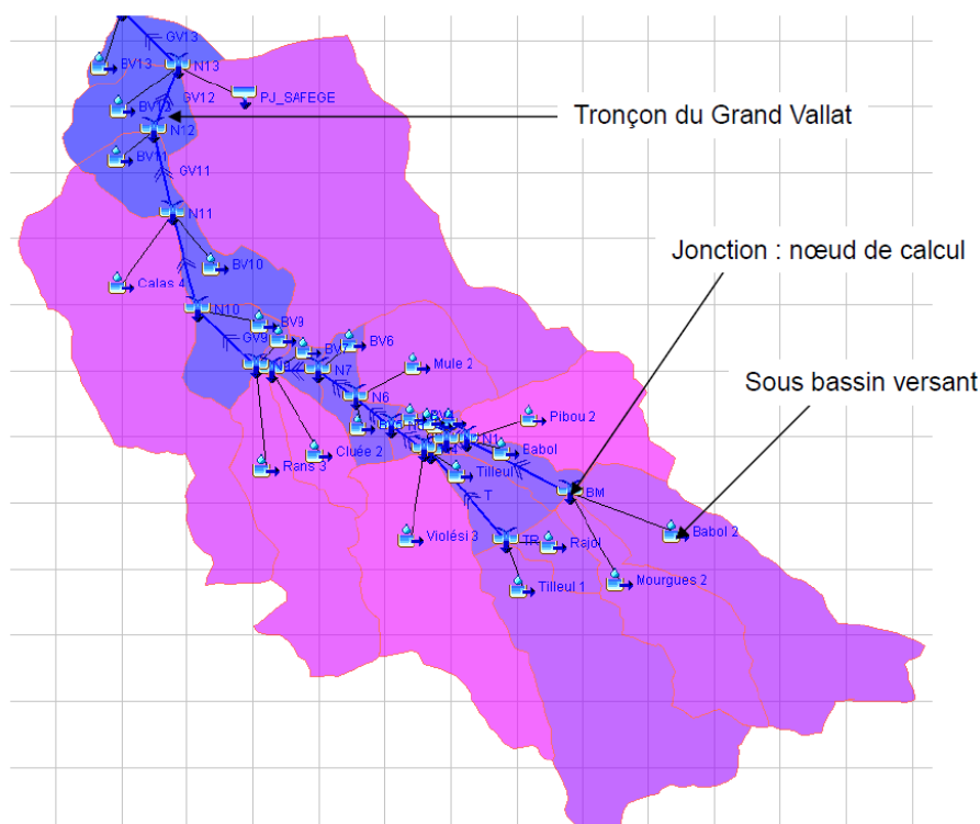
Figure 13 : Modèle Pluie-Débit HEC-HMS (source : Etude pour la réduction de l'aléa inondation au droit des lieux habités en tenant compte du fonctionnement naturel des cours d'eau sur le bassin versant de la Jouïne et du Grand Vallat, INGEROP– SABA, 2013)
