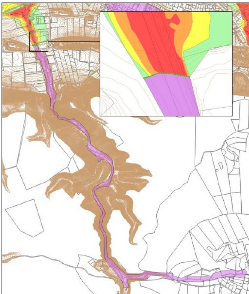
Figure 41 : Précision de l'aléa : Vallat des Tilleuls (DDTM-INGEROP-2018)
