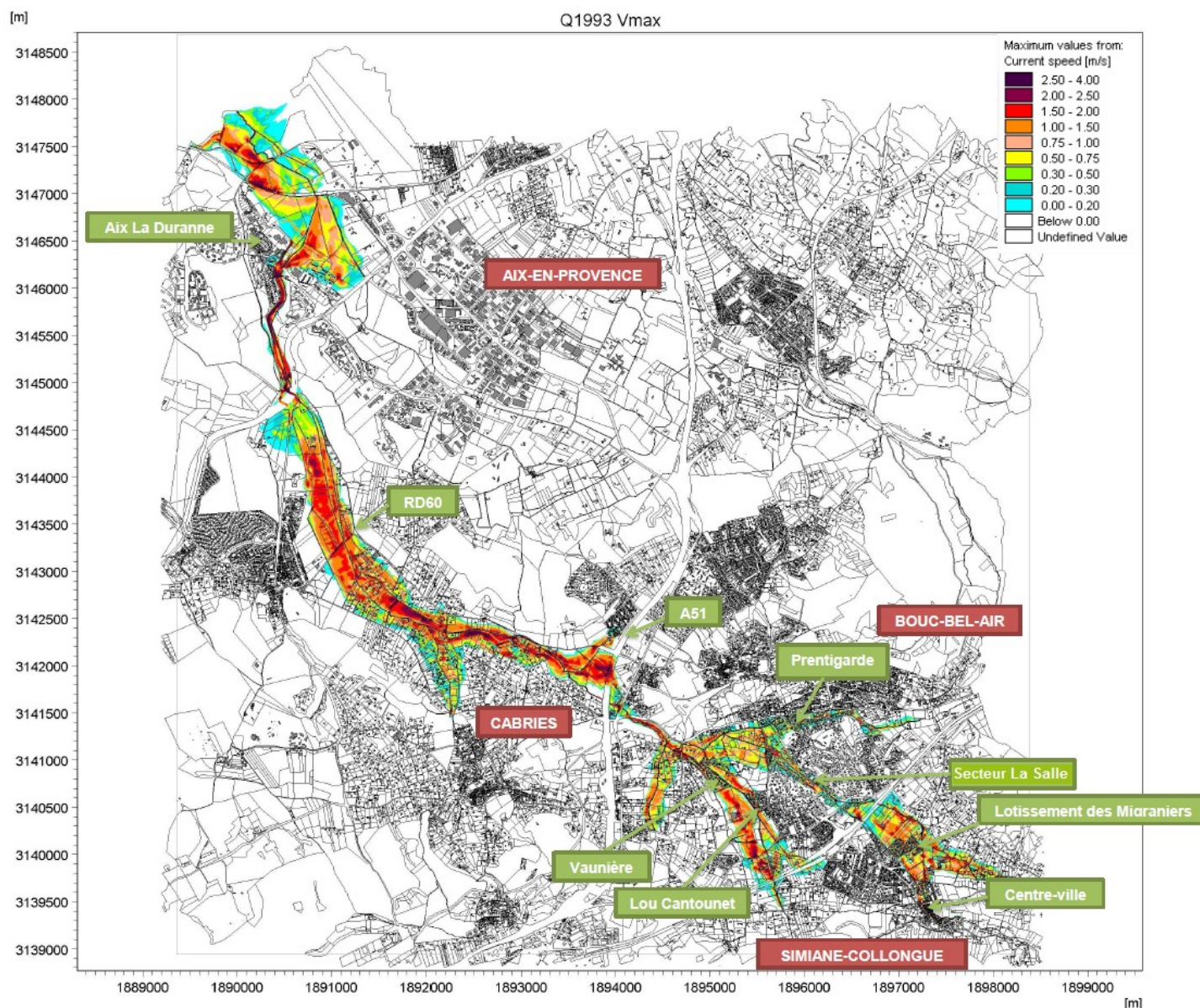
Figure 22 : Vitesse pour l'événement de référence, Q1993 (Source INGEROP – SABA, 2013)
