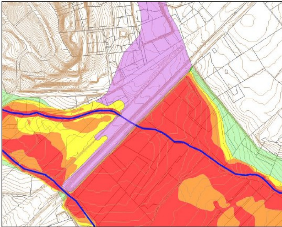
Figure 36 : Précision de l'aléa : Vallat de Babol – secteur 2(DDTM-INGEROP-2018)
