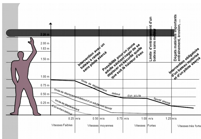
Figure 45 : Mobilité en terrain inondé en fonction de la vitesse et de la hauteur d'eau
