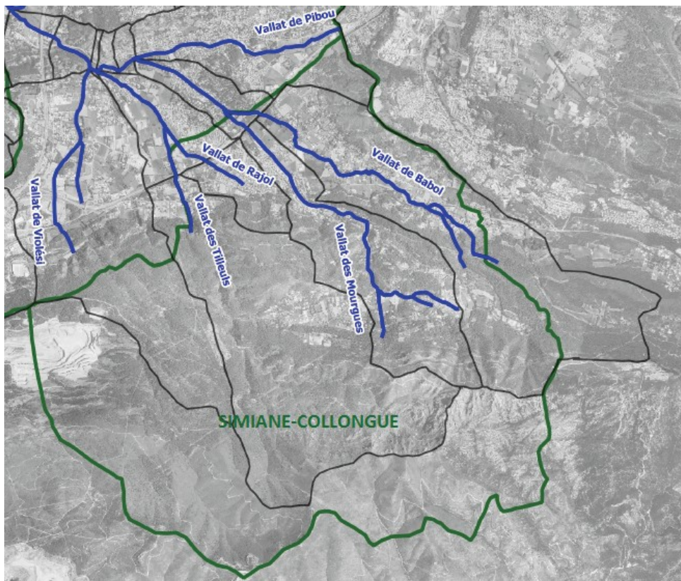
Figure 3 : Zoom sur la commune de Cabriès : Cours d'eau concernés par l'étude pour la réduction de l'aléa inondation au droit des lieux habités en tenant compte du fonctionnement naturel des cours d'eau (Bassin versant Jouïne – Grand Vallat)
