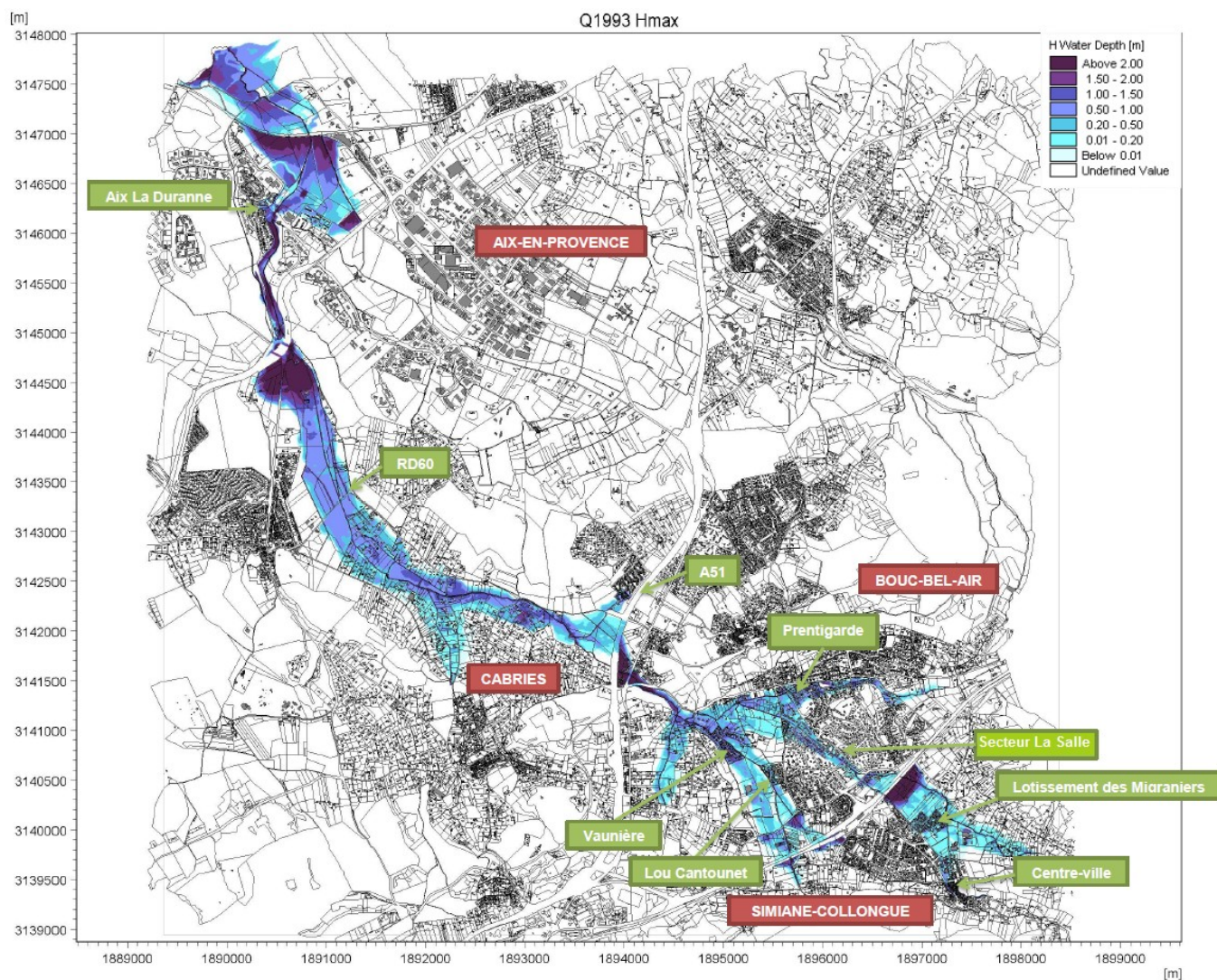
Figure 21 : Hauteurs d'eau pour l'événement de référence, Q1993 (Source INGEROP – SABA, 2013)
