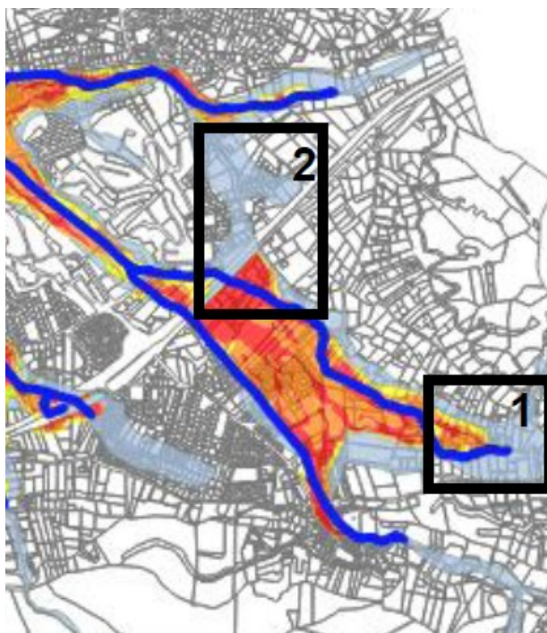
Figure 32 : Localisation des secteurs étudiés le long du Vallat de Babol sur la commune de Simiane-Collongue (DDTM-INGEROP-2018)
