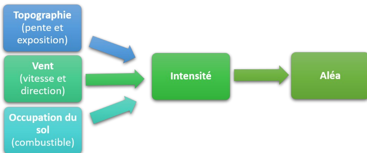
Figure 2: Diagramme de construction de l'aléa subi
