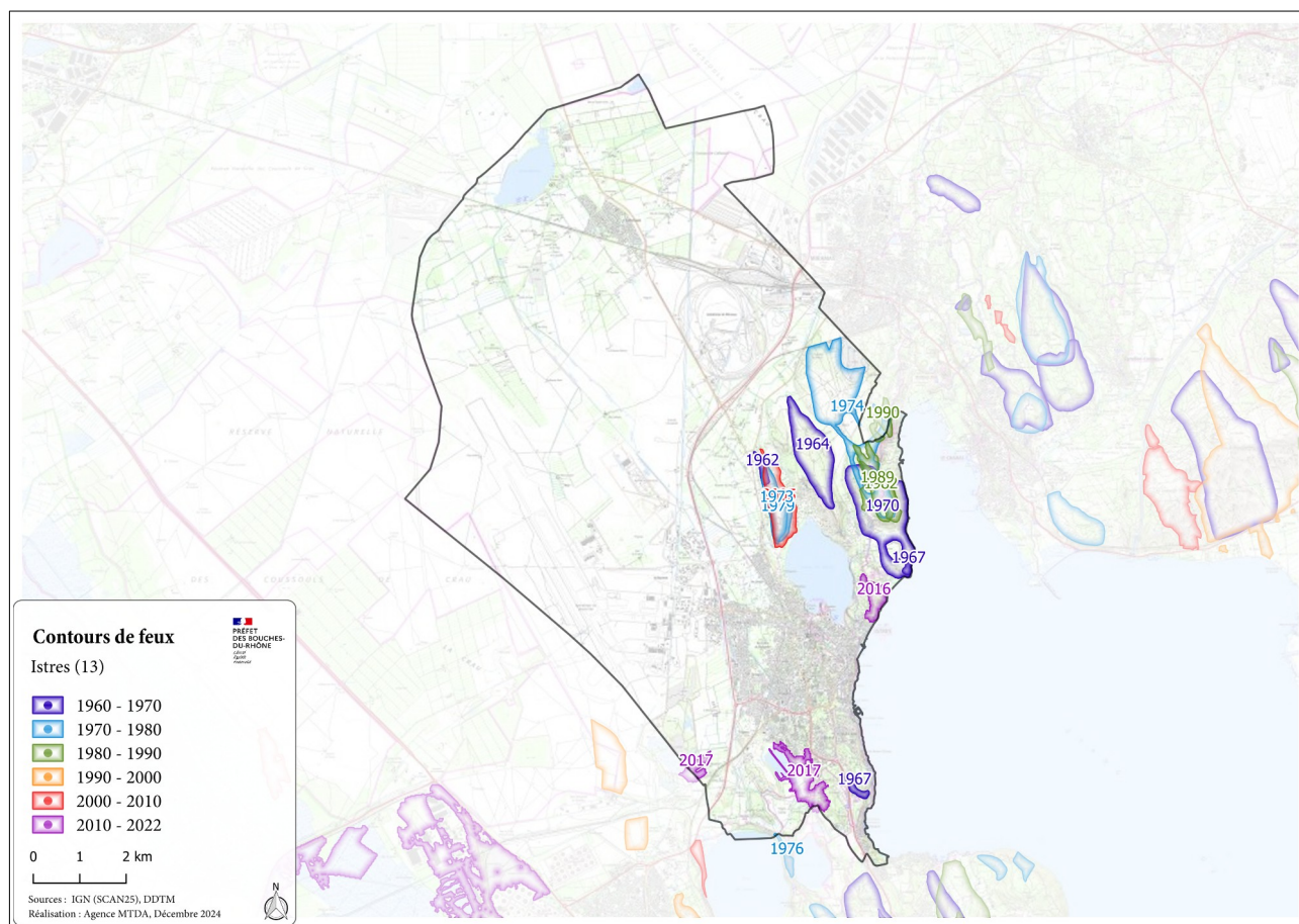
Illustration 8 : Carte des contours des feux d'Istres
