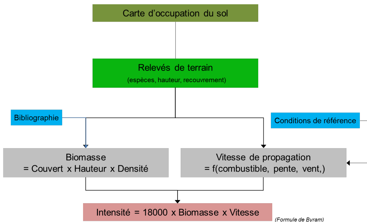
Illustration 14: Etapes de modélisation du combustible
