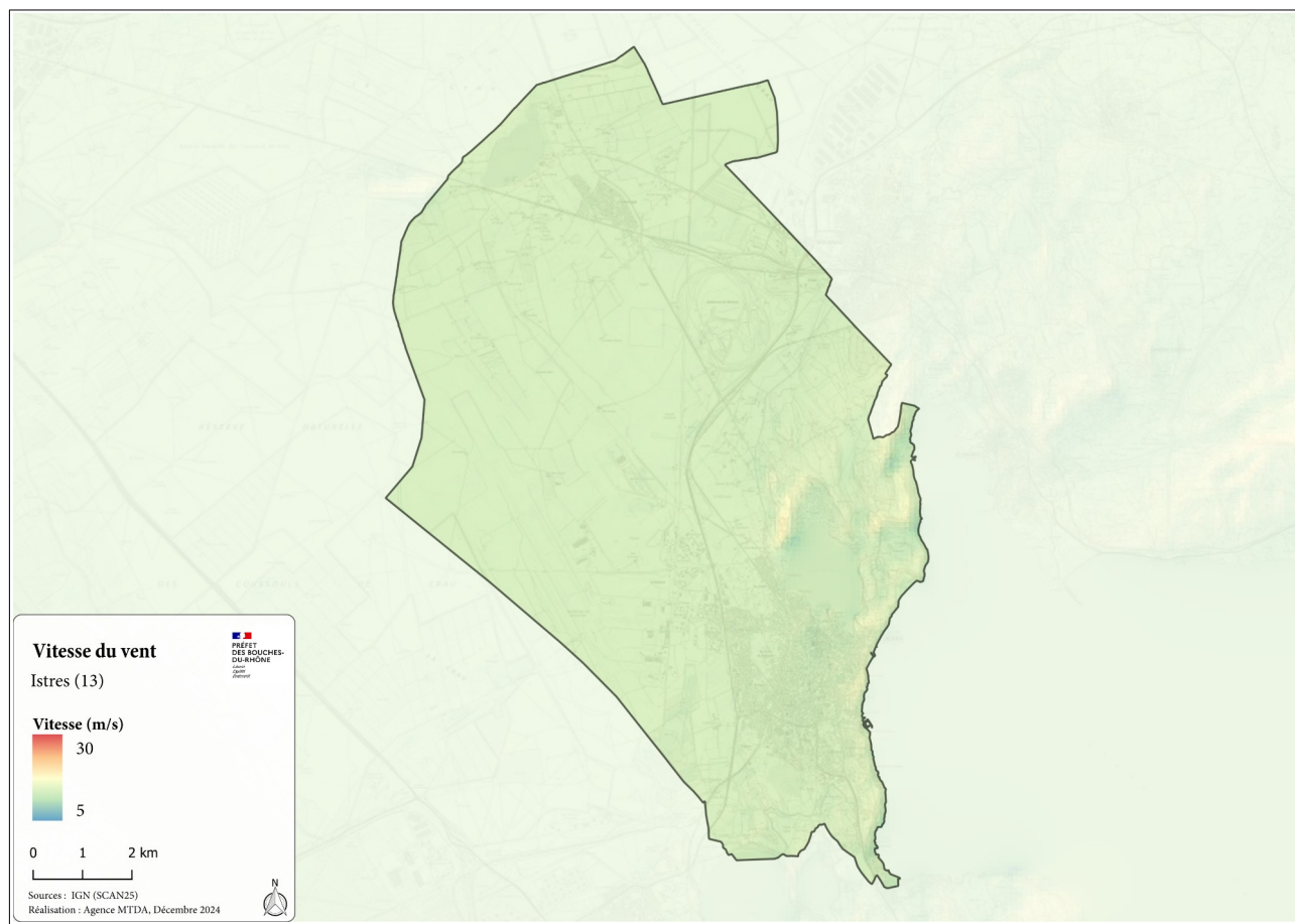
Illustration 7 : Carte des vitesses du vent d'Istres
