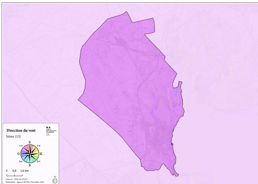
Illustration 6 : Carte des directions du vent d'Istres
