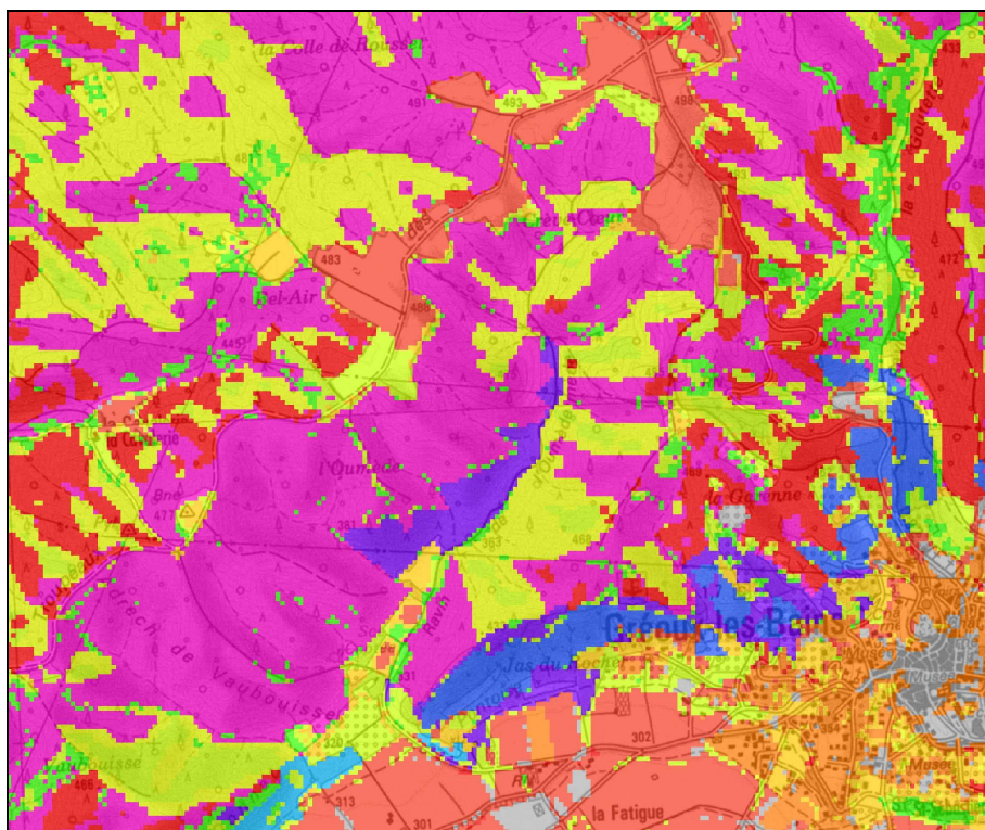
classification supervisée
