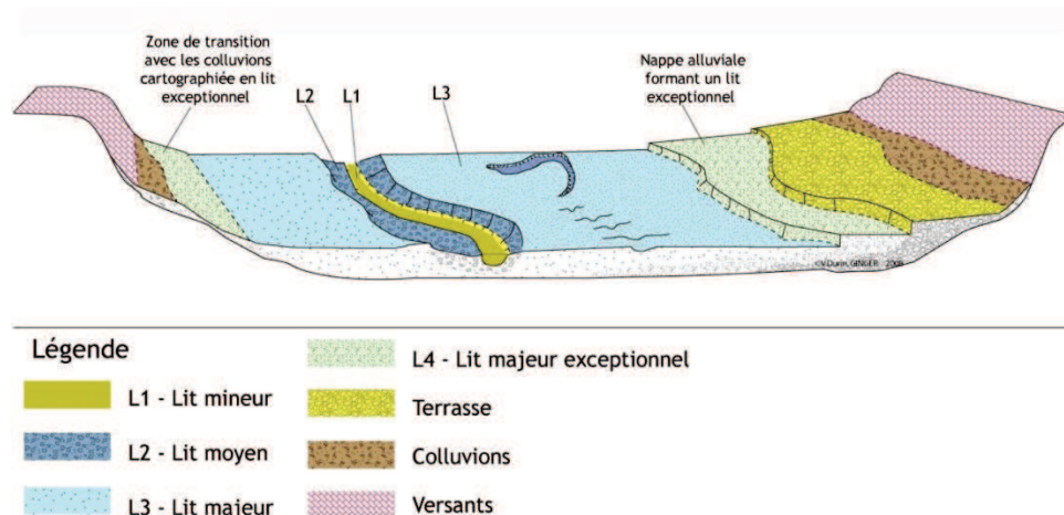
Illustration 10 - Morphologie d'un cours d'eau
