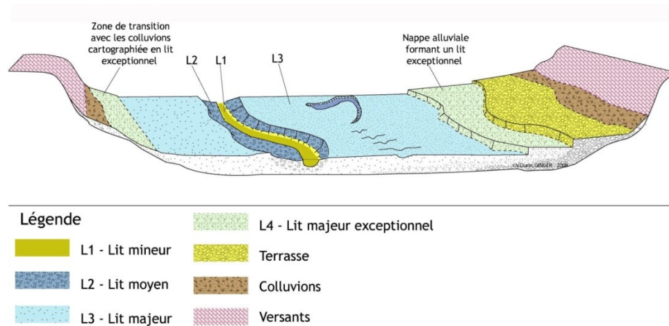
Illustration 14 - Morphologie d'un cours d'eau
