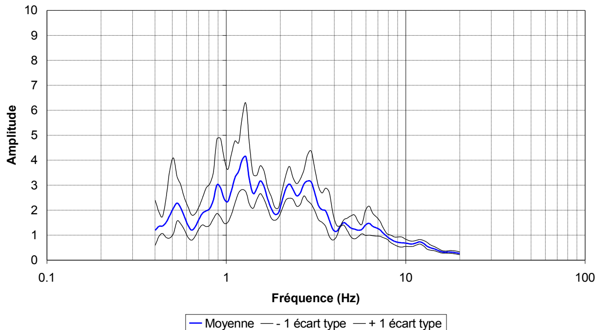
Figure 12 : Fonction de transfert du site GBGA, estimée par la méthode H/V sisme (enregistrement du séisme des Saintes, 21/11/2004).
