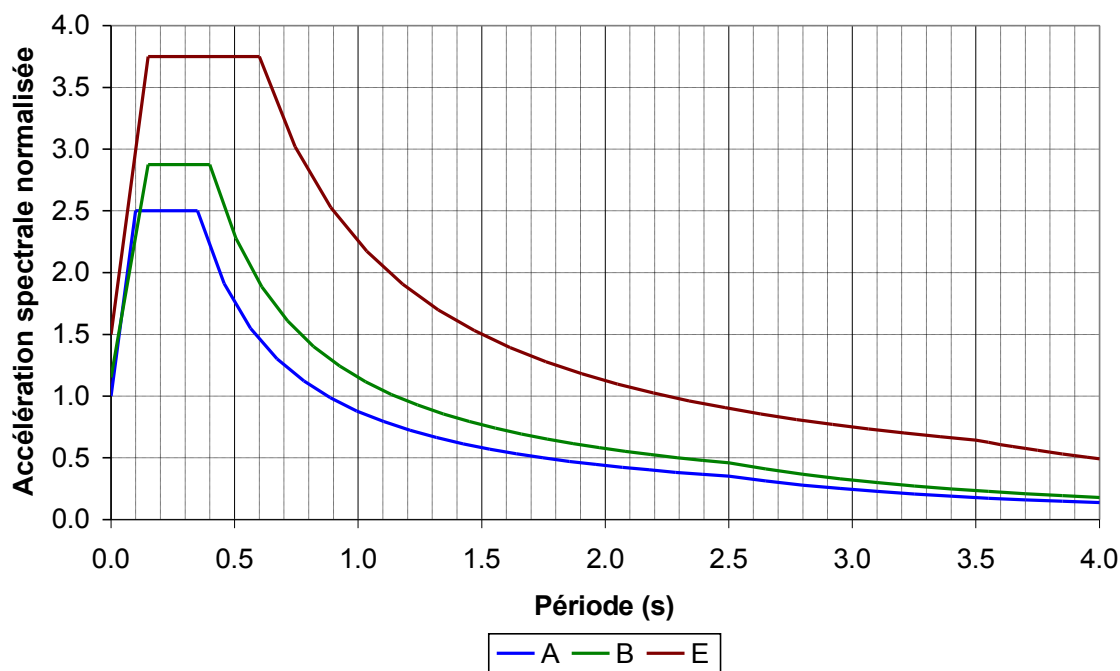
Figure 19 : Spectres de réponses normalisés associés aux différentes zones présentant une réponse sismique homogène
