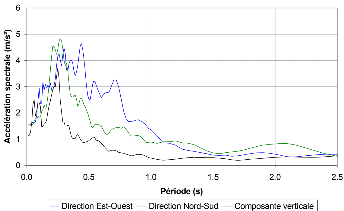
Figure 11 : Spectres de réponse de l'enregistrement du séisme des Saintes (21/11/2004) à Marie-Galante.
