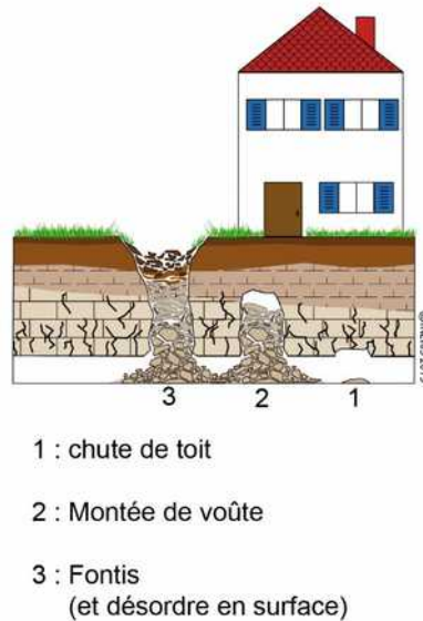
Figure 16 : Principe du fontis initié par une chute de toit
