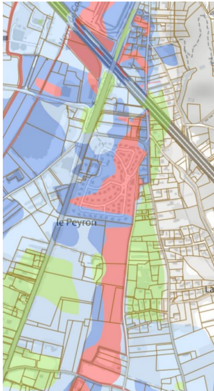
Carte 4 : Extrait de la cartographie des aléas du PPRI modifié - secteur Peyron
