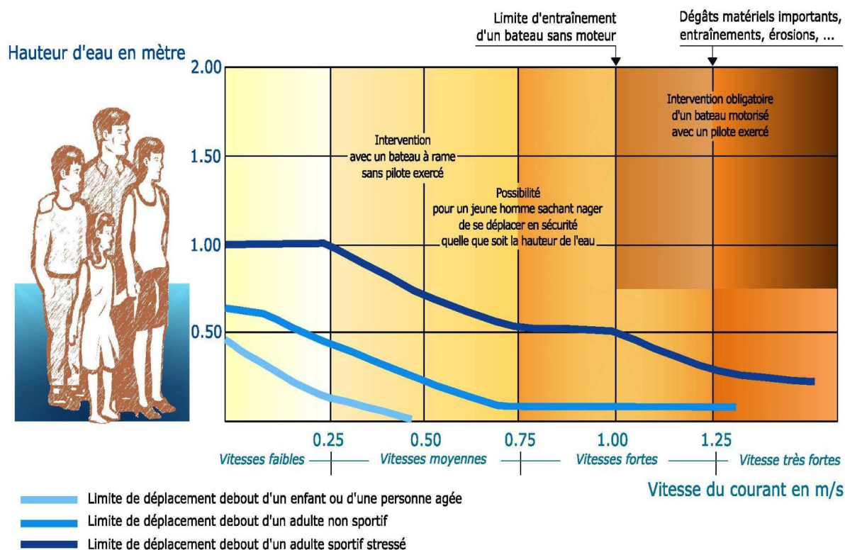
Illustration 15: Grille de danger de l'eau selon sa hauteur et sa vitesse
