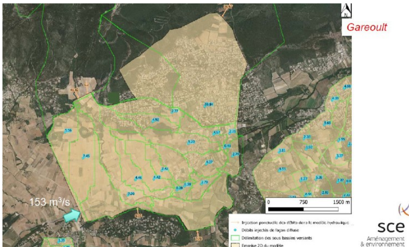
Illustration 10: Débits de pointe des hydrogrammes injectés dans les modèles hydrauliques sur Garéoult
