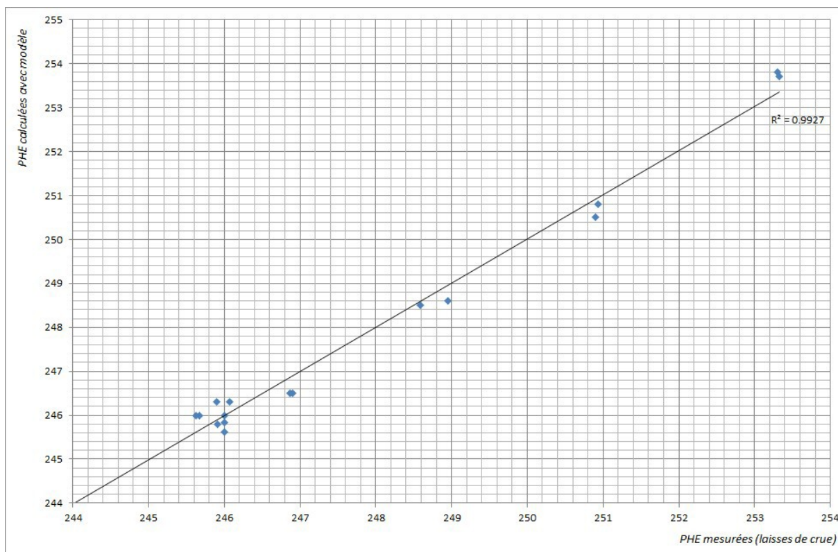
Illustration 13: Comparaison entre PHE mesurées et calculées sur le territoire de Besse sur Issole pour une crue comparable à celle de janvier 1999.
