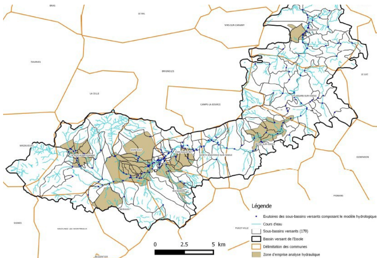
Illustration 8: Unités hydrographiques retenues pour le développement du modèle Pluie-débit avec emprise indicative des modèles hydrauliques.
