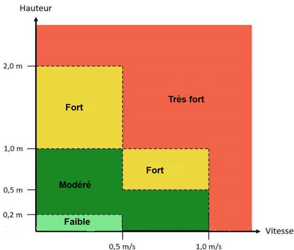
Illustration 16: Grille d'aléa du PPRI
