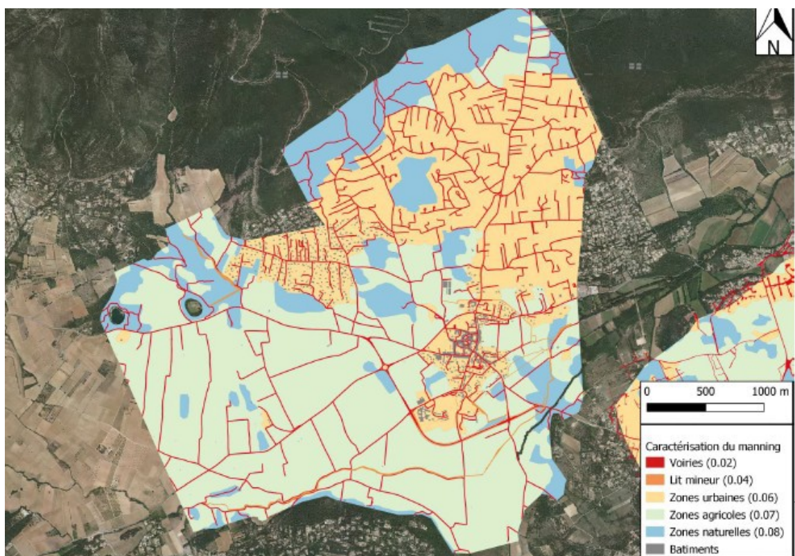
Illustration 14: Coefficient de rugosité retenus sur Garéoult
