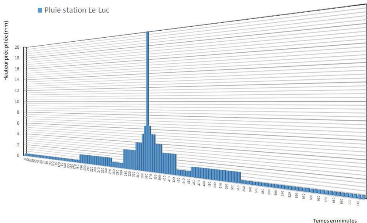
Illustration 7: Hyétogramme de pluie de référence obtenu par agrégation des hauteurs de référence de pluie.
