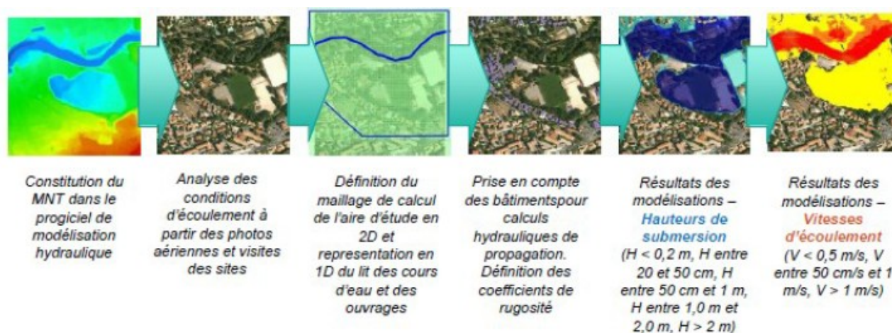
Illustration 11: Etapes de construction et d'exploitation d'un modèle hydrauliques
