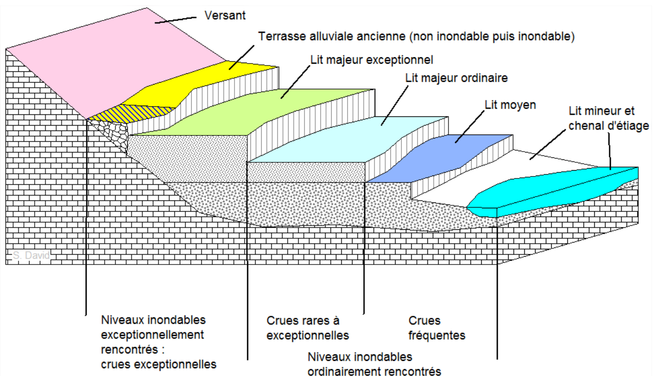
Illustration 5: Représentation schématique de l'empilement normal des unités hydrogéomorphologiques
