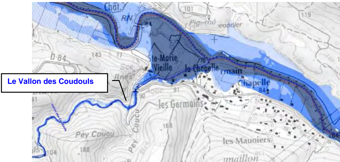
Figure 29: Hauteurs d'eau et vitesses d'écoulement – L'Argens
