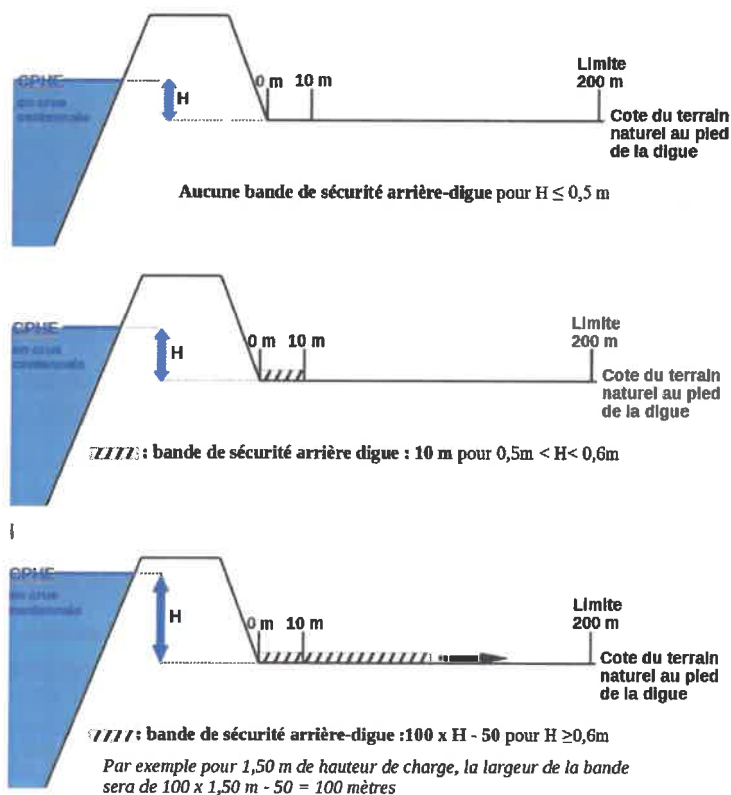
Figure 23 : Délimitation des bandes de sécurité arrière-digue.
