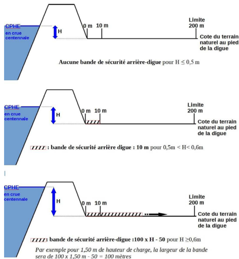
Figure 23 : Délimitation des bandes de sécurité arrière-digue.
