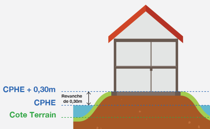
Figure n°7 : Illustration de l'implantation d'un bâtiment au-dessus de la CPHE + 0,30 m. Source : Mayane pour la DDT du Bas-Rhin, 2018.
