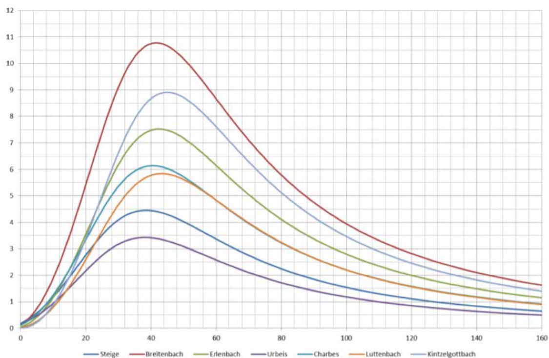
Figure 17 : Hydrogrammes des affluents du Giessen estimés et utilisés pour le PPRI.
