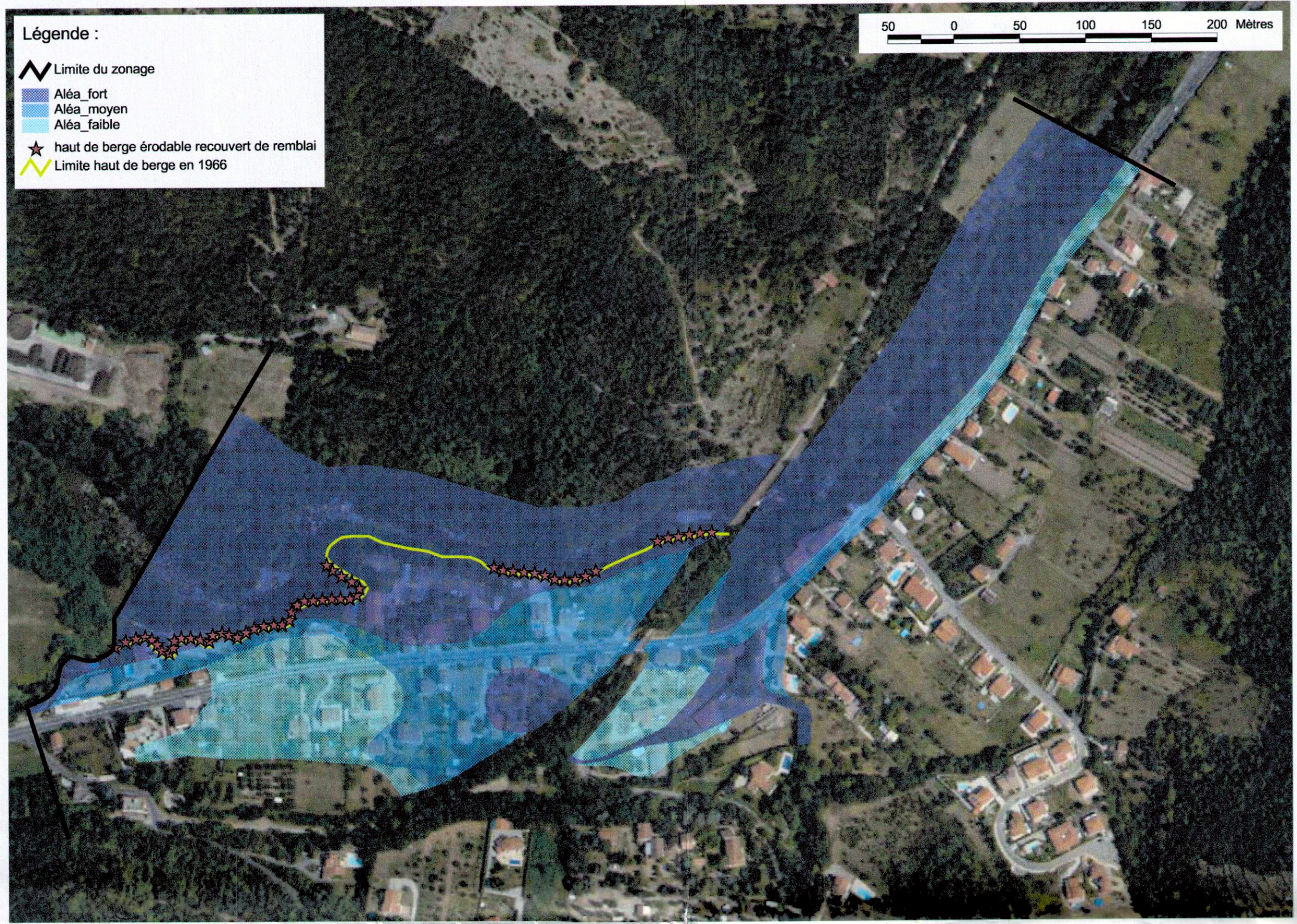
Expertise hydraulique complémentaire pour la détermination de l'aléa inondation - Secteur de la Forge - RTM 2012
