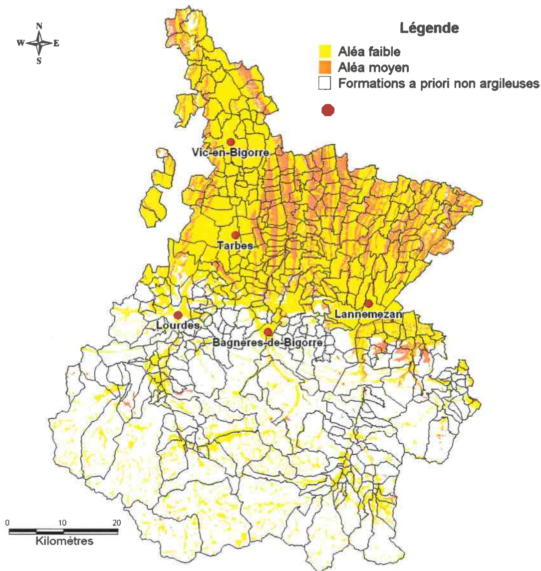
III. 3 : Carte d'aléa retrait-gonflement des argiles dans le département des Hautes-Pyrénées
