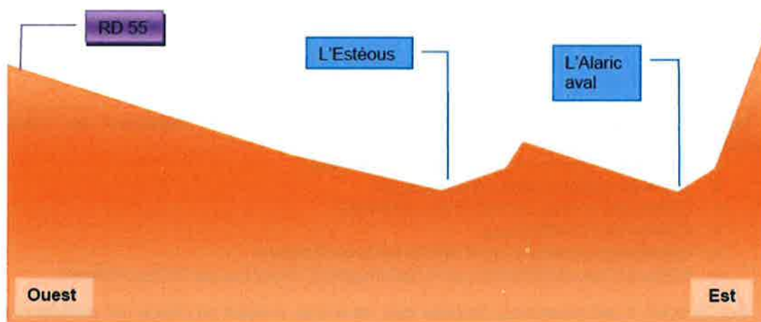
Profil géomorphologique schématique en amont de Sauveterre
