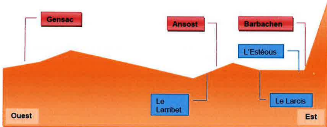
Profil géomorphologique schématique au niveau de Barbachen
