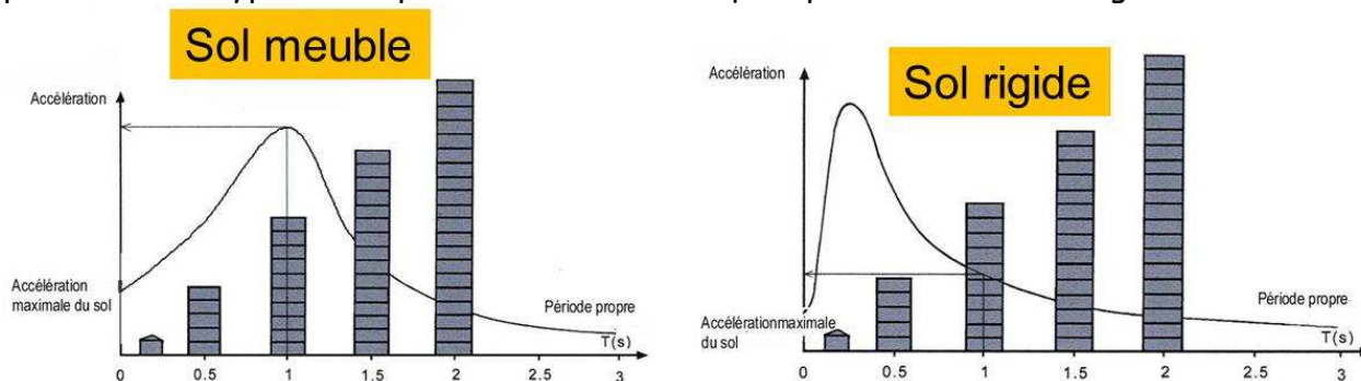
Figure 10 : Spectre de réponse des sols et période de résonance de bâtiment. Les immeubles élevés (ou souples) subissent une agression plus forte sur des sols meubles. A l'inverse, les effets de site associés à des sols rigides agressent plus nettement des constructions de faible hauteur.
