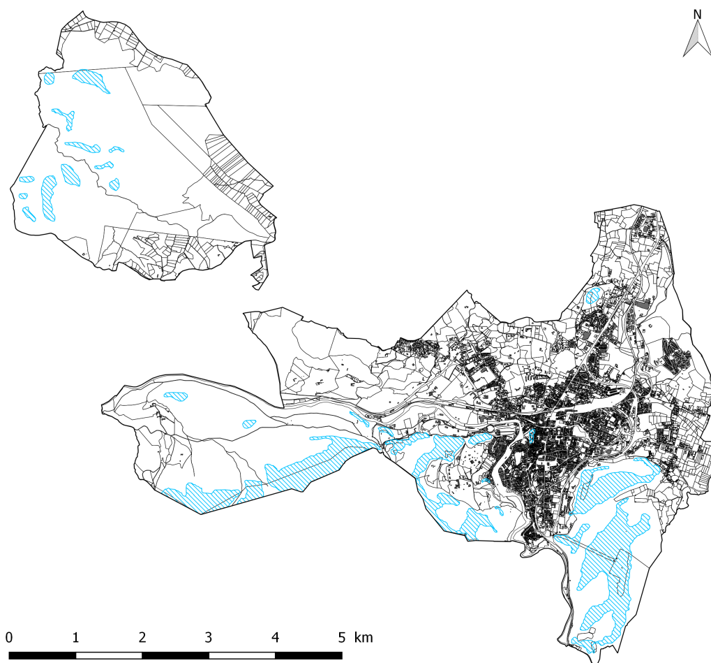
Figure 13 : Zones susceptibles de présenter un effet de site topographique sur la commune de Lourdes (d'après Bernardie et al., 2006).
