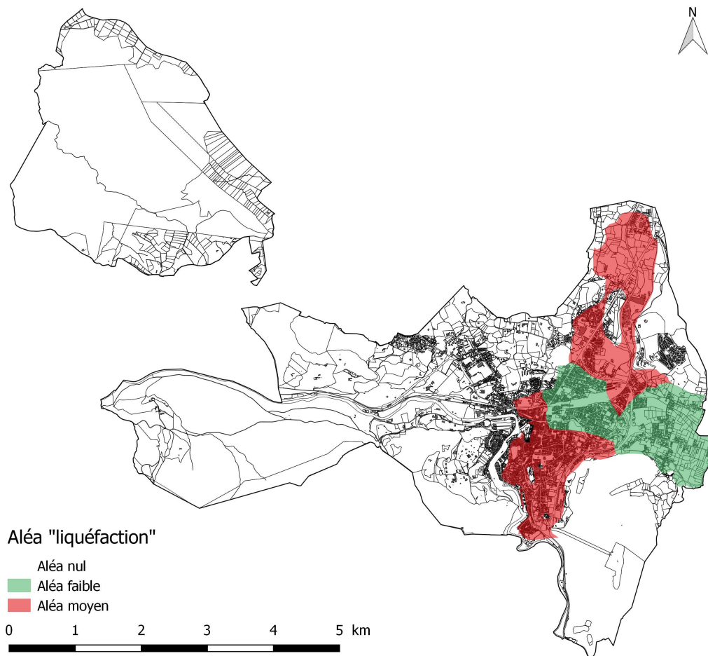
Figure 14 : Cartographie de l'aléa liquéfaction sur Lourdes.
