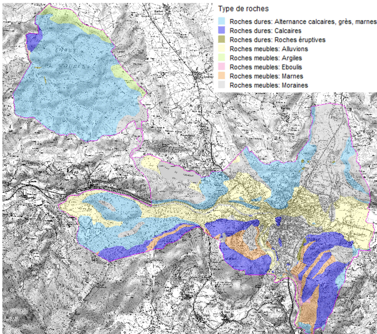
Figure 4 : Type de roches sur la commune de Lourdes sur fond topographique (d'après la carte géologique de la feuille n° 1052 de Lourdes 1/50 000 - BRGM )
