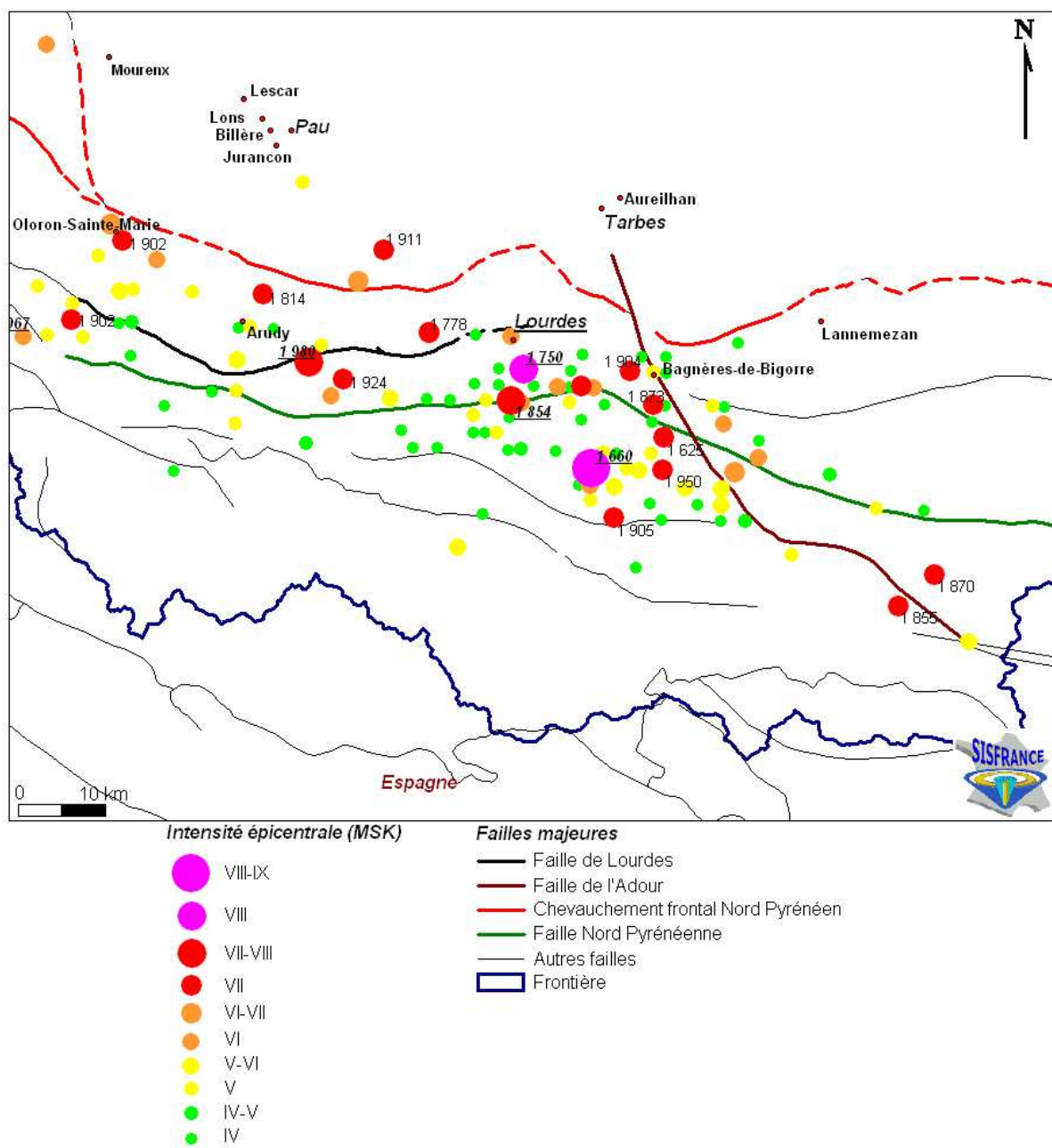
Figure 5 : Sismicité historique de la région de Lourdes (base de données SisFrance, BRGM-EDF-IRSN, www.sisfrance.net ) et localisation des failles.
