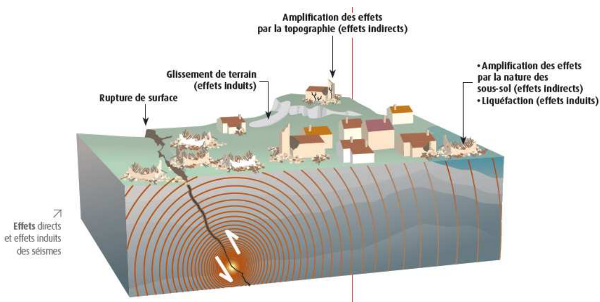
Figure 7 : Aléa sismique local
