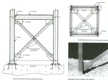
exemple de contreventement
