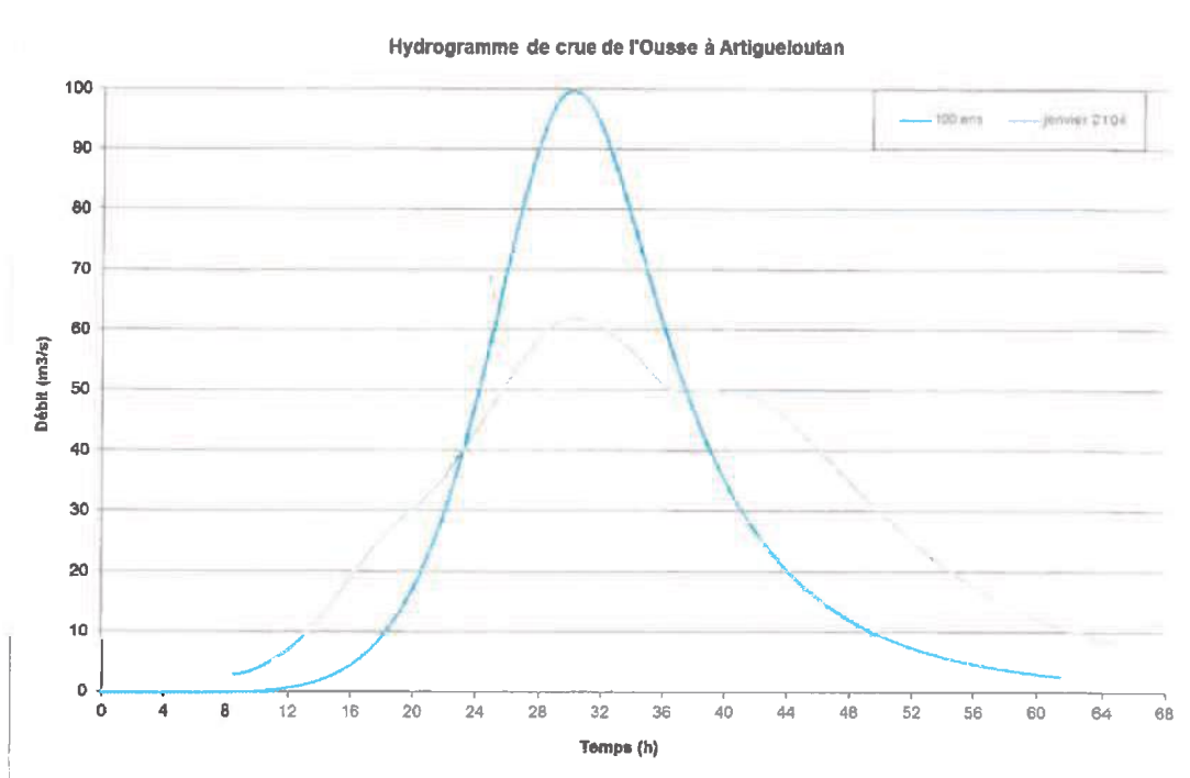
Figure 29 : hydrogrammes de crue théorique et modèle de janvier 2014
