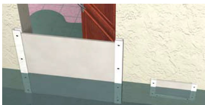
Batardeau de porte et couverture d'entrée d'air limitant la pénétration de l'eau
