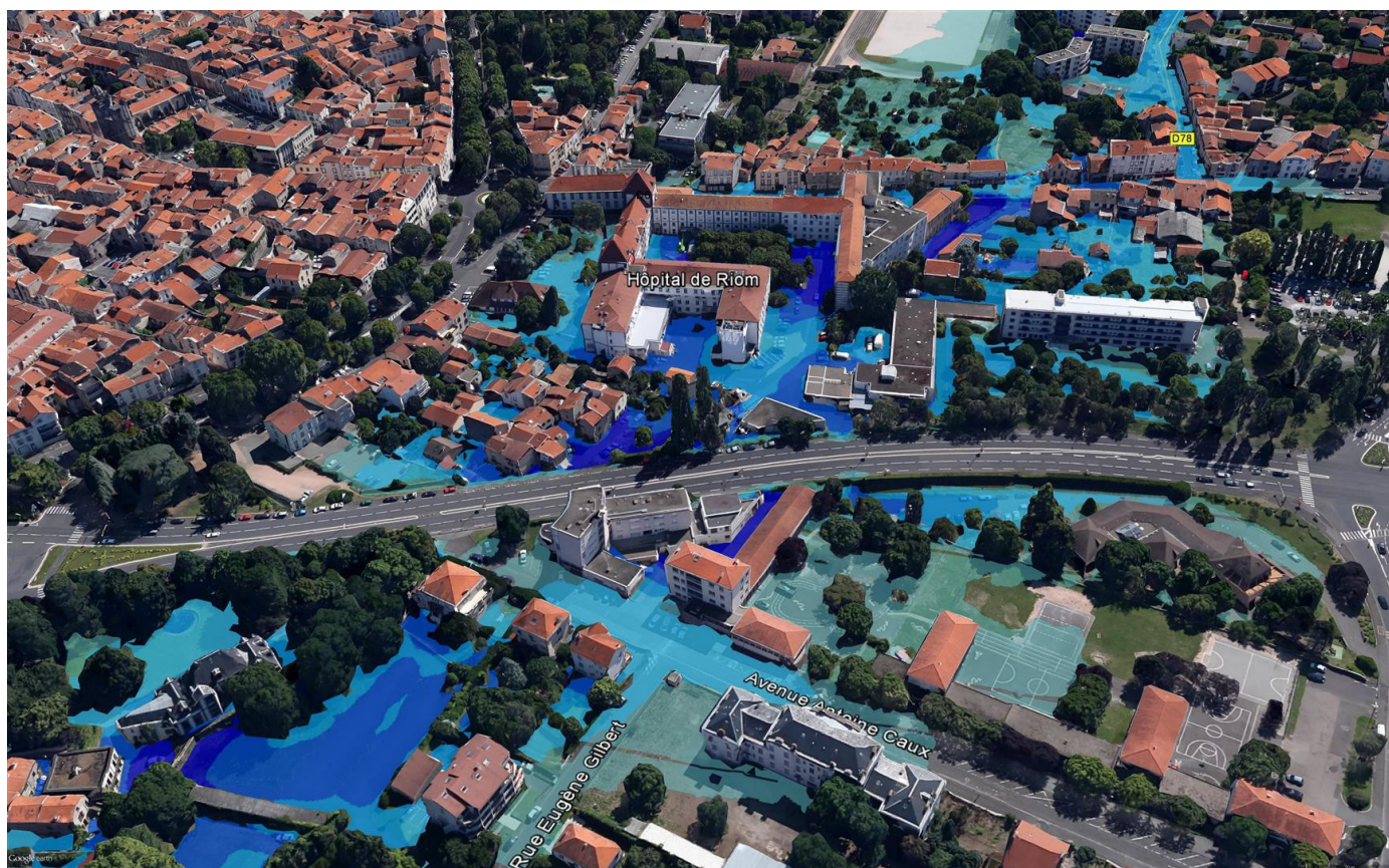
Reconstitution en 3D des hauteurs d'eau dans le secteur de l'hôpital de Riom
