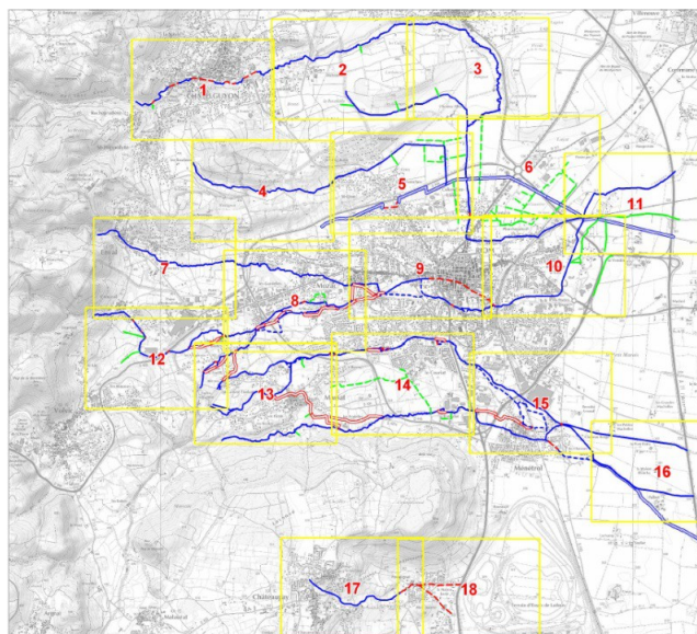
Illustration de levés d'ouvrages d'art et profils en long des cours d'eau
