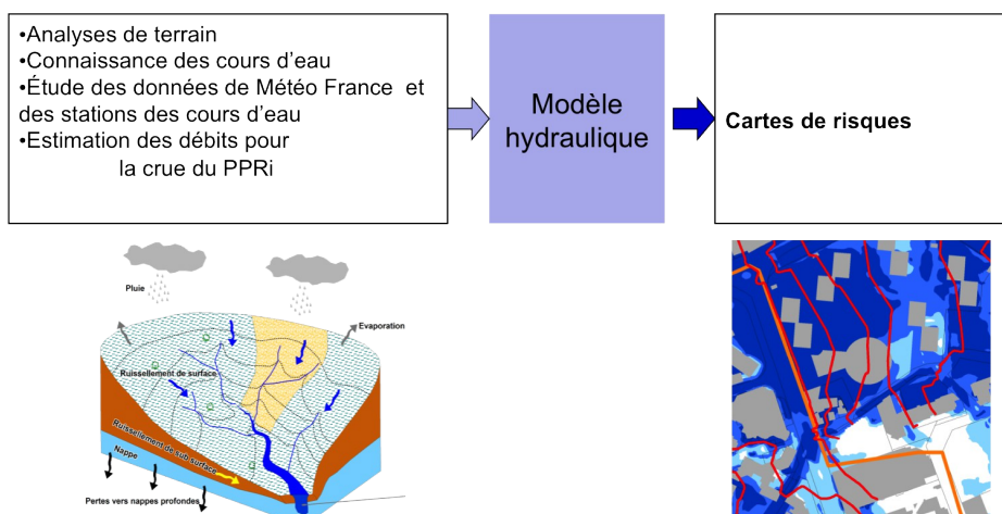
Principe de l'étude de modélisation hydraulique de 2014
