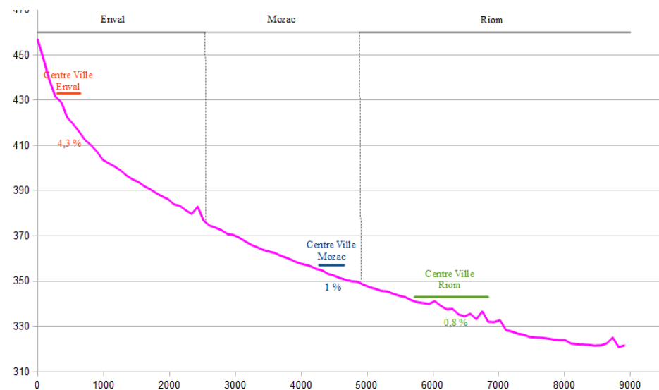
Illustration des types d'écoulement sur l'Ambène (représentation du profil en long de la rivière)
