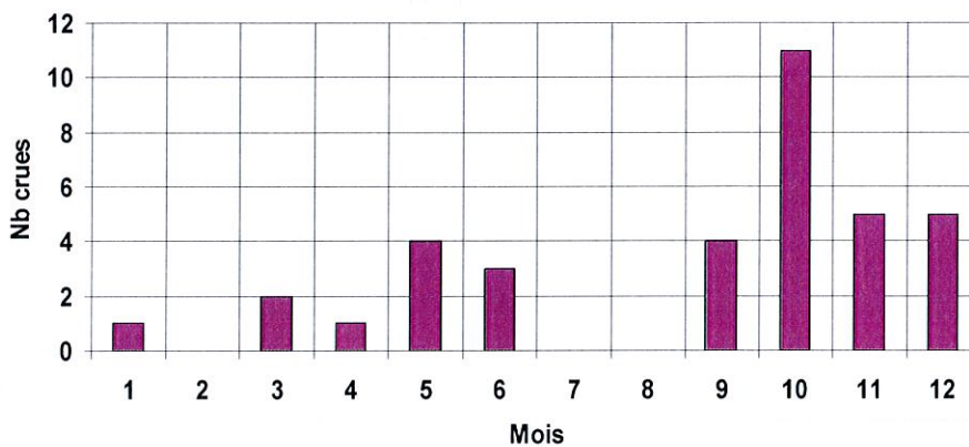
Nombre de crues entre 1835 et 2010 dont la hauteur à Vic le Comte a dépassé 3 m ou dont le débit a dépassé 700 m 3 /s
