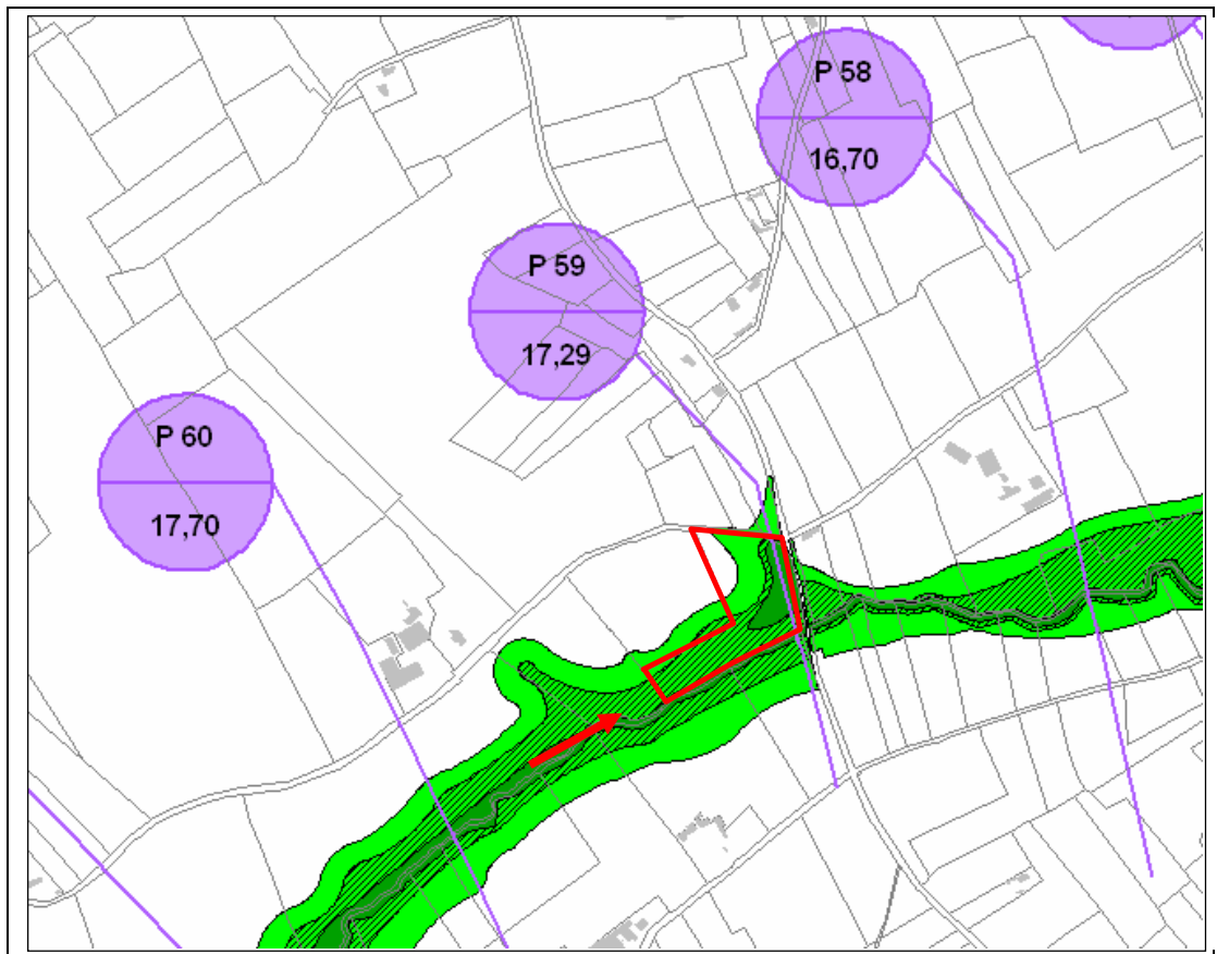
Schéma de principe de définition de la cote de crue centennale au droit de la parcelle aménageable entourée de rouge
