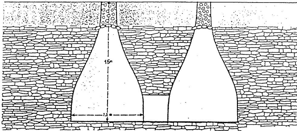
Coupe des exploitations dites en bouteilles
