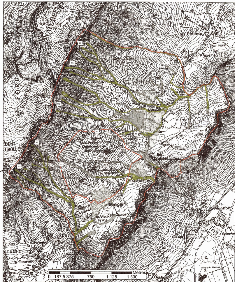
Carte des aléas "crues des torrents et des ruisseaux torrentiels" et "ruissellements sur versants" Echelle : 1/10000 (fond IGN Scan EDR)
