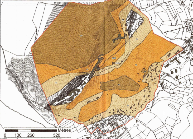
Carte des aléas "mouvements de terrain" sur le versant dit des "Etablissements Hospitaliers" Echelle : 1/5000 (fond topographique et cadastral)
