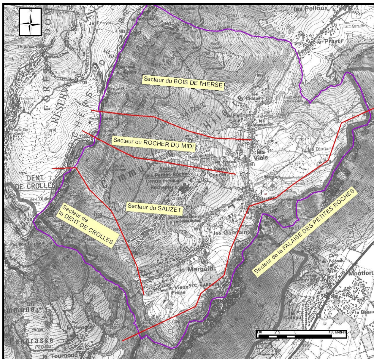
Figure n°15: Carte des secteurs de chutes de blocs (fond : scan 25 IGN, 2001)
