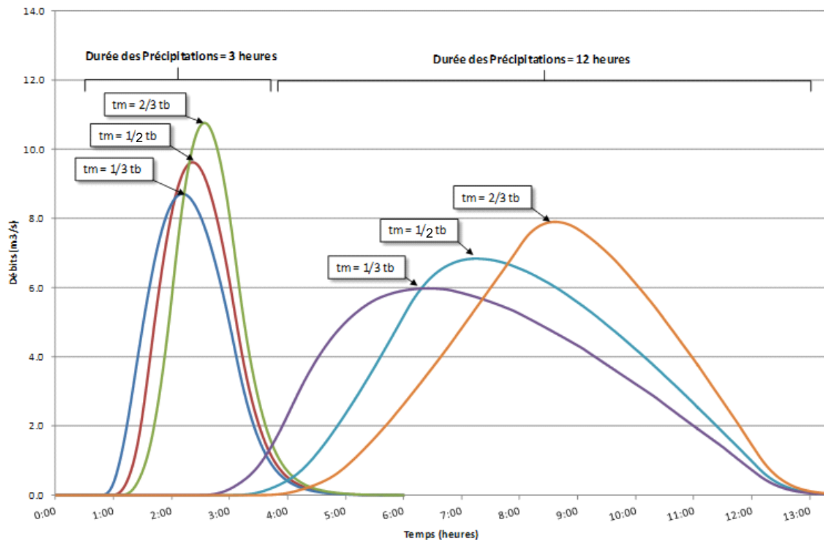
Illustration 6 : les 6 hydrogrammes retenus pour la modélisation du Charmeyran
