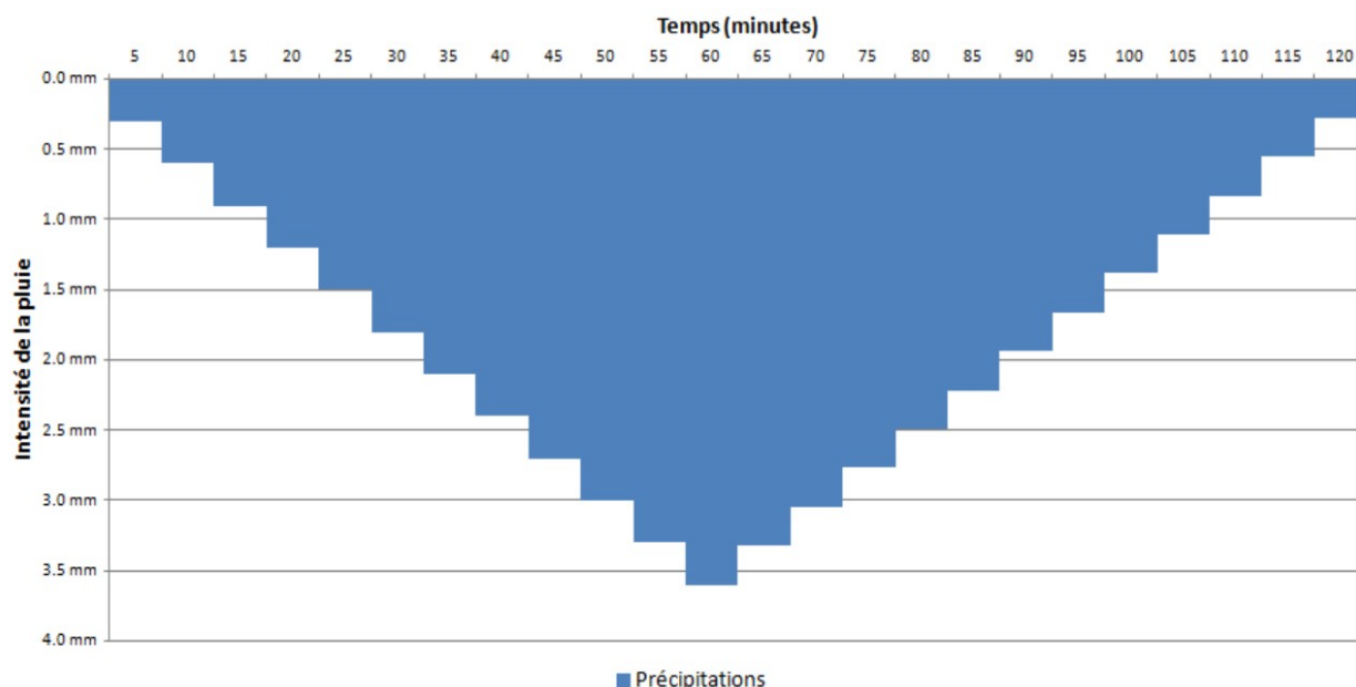
Illustration 11 : hyétogramme retenu pour la modélisation
