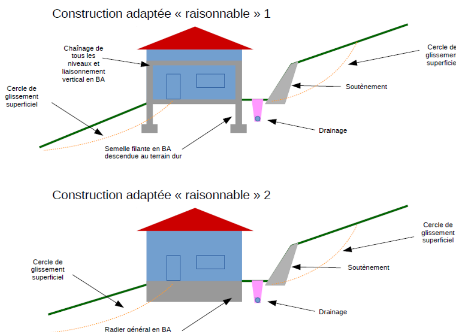
Illustration 15 : schéma d'un bâti adapté à l'aléa de glissement de terrain
