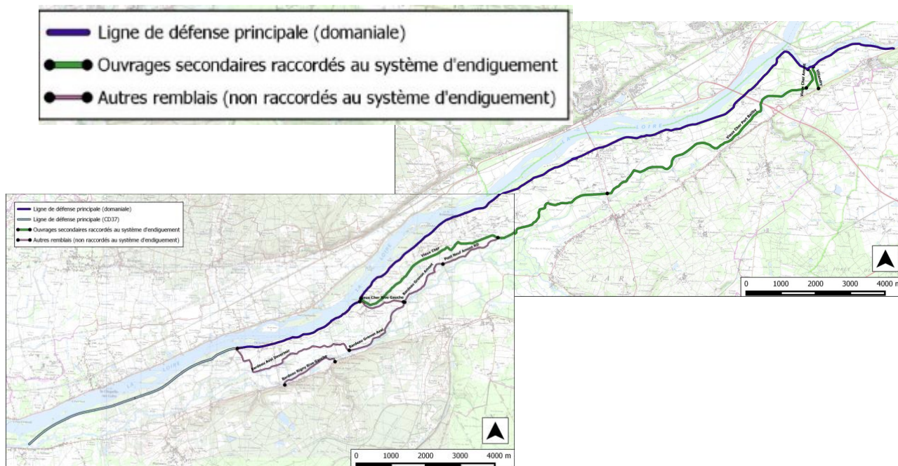
Système d'endiguement du Val de Villedry/Bréhémont
