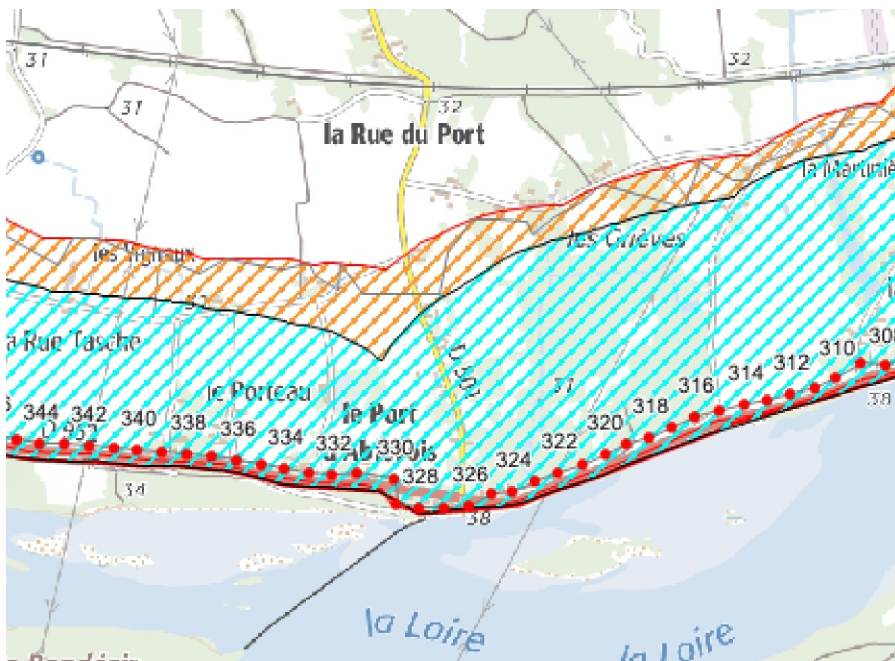
Extrait : représentation des profils CardDiques pour calcul de la ZDE tenant compte des longueurs de brèche (moyenne calculée sur 400 m) – délimitation brute de la ZDE en orange, et délimitation moyennée en bleu
