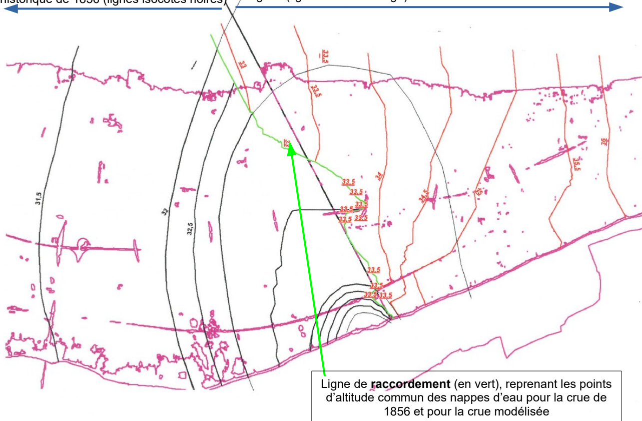
Raccordement des deux nappes d'eau (crue de 1856, crue modélisée T200)
