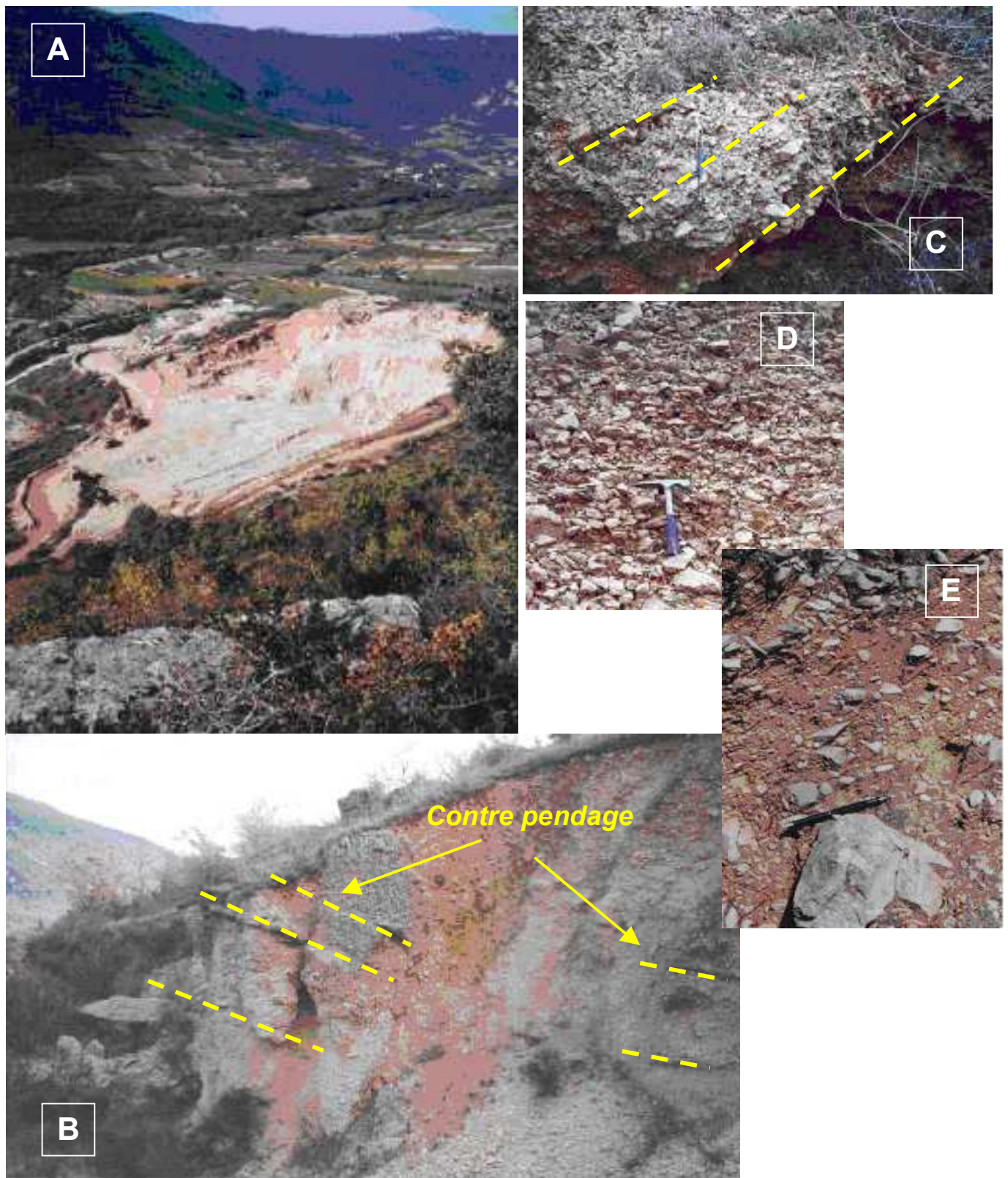
Figure 12 : Formation de Versant : A : formations de versant exploitées par la carrière de Baldares. Notons l'importance de l'épaisseur et de l'étendu de ces formations.; B : éboulis de pente non consolidés constitués d'éléments plus ou moins anguleux, emballés dans une matrice limoneuse à argileuse plus ou moins abondante. Notons le contre-pendage que présentent ces formations ; C : éboulis de pente consolidés. Notons également le contre-pendage.; D : éboulis de pente à matrice très réduite; E : éboulis de pente emballés dans une abondante matrice limoneuse.
