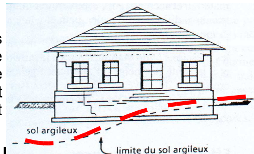
Figure 37 : Exemple de désordres sur une construction dus à la variation d'épaisseur du sol argileux sensibles.
