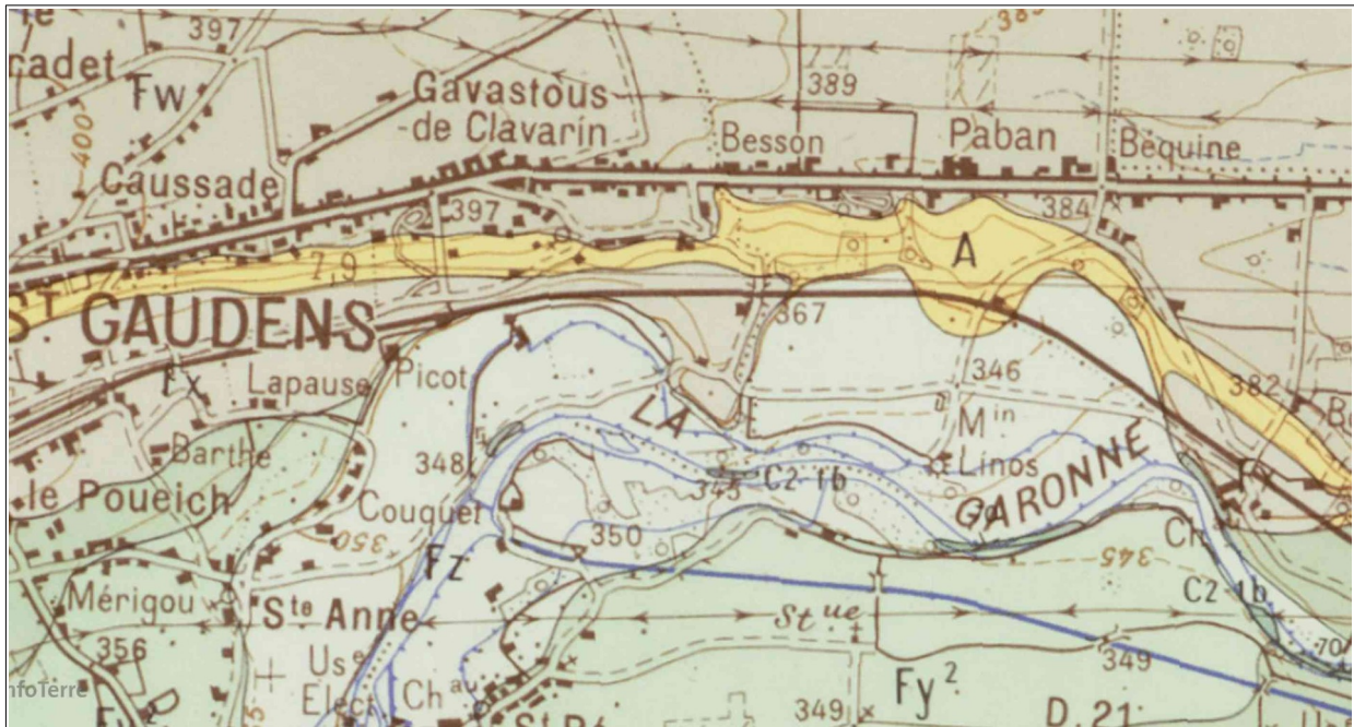
Figure n° 26 : extrait de la carte géologique BRGM au 1/50 000 de la commune de Saint-Gaudens sur le secteur des Gavastous
