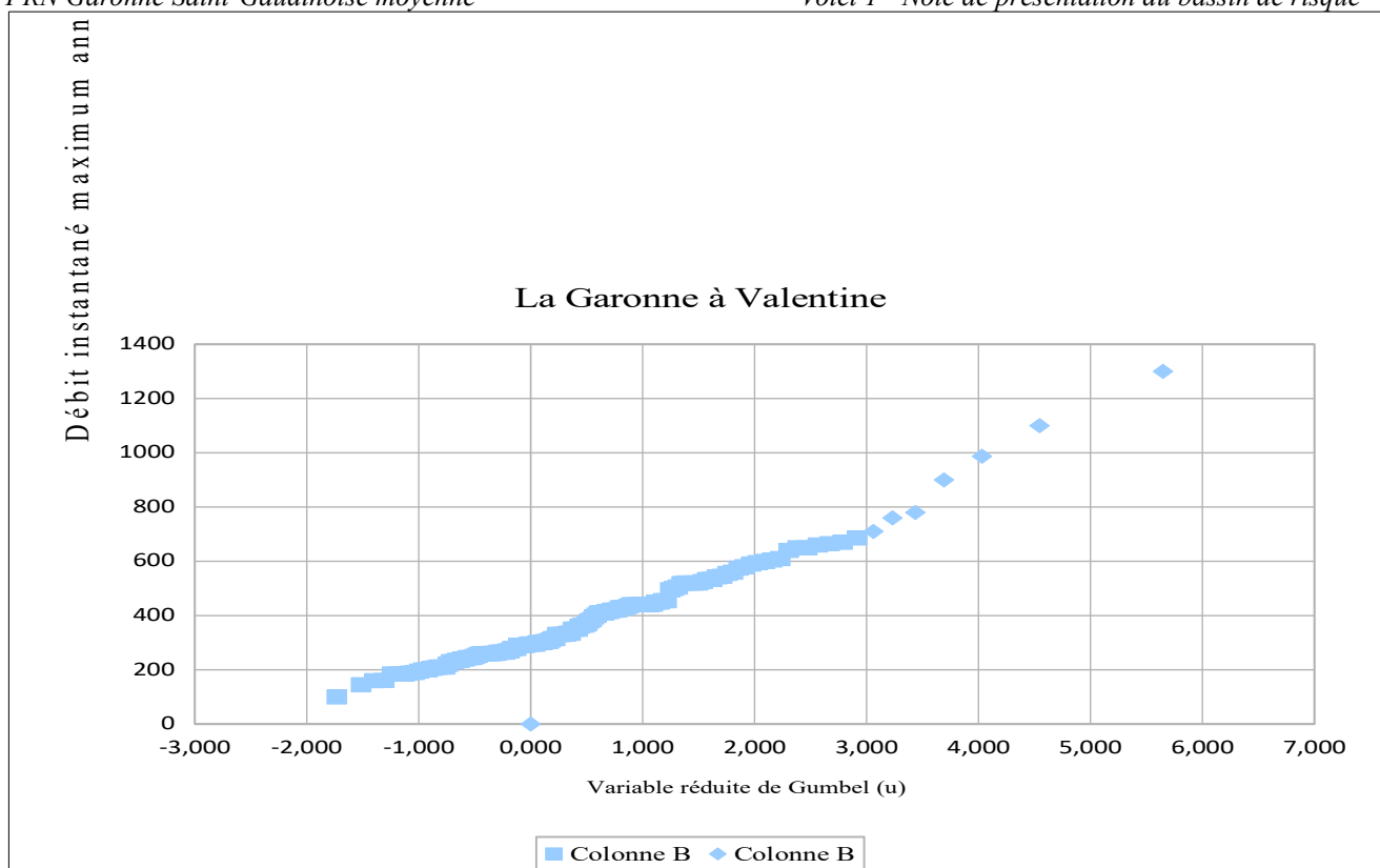
Figure n° 8 : graphique de la période de retour de la Garonne à Valentine
